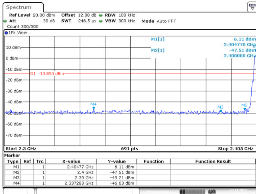
Zigbee_Ant1_Low_2405MHz
