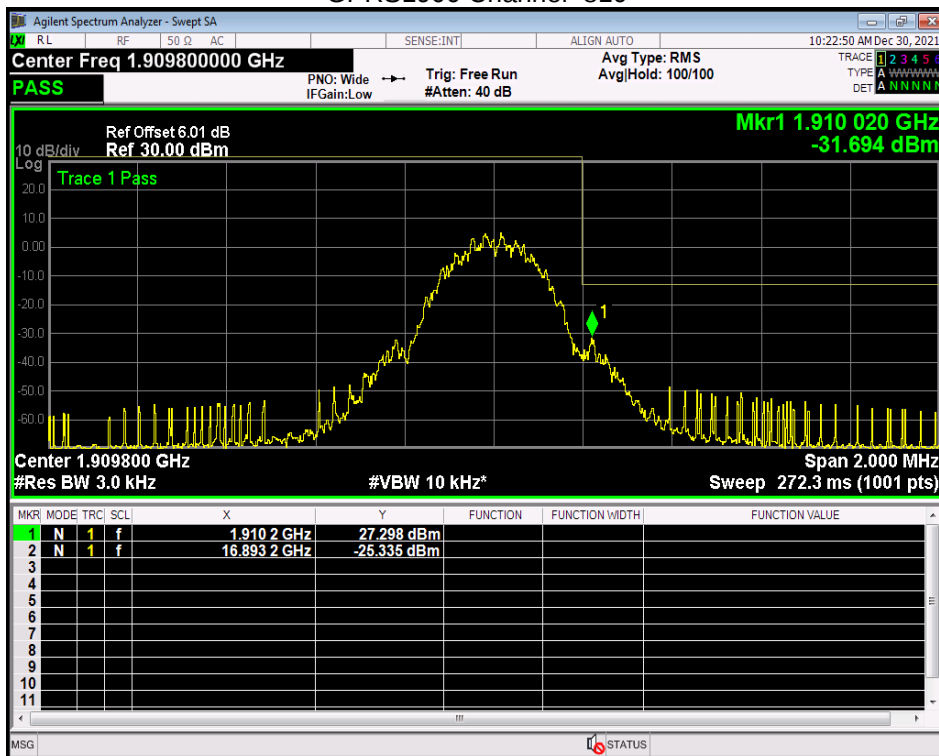
GPRS1900 Channel=810
