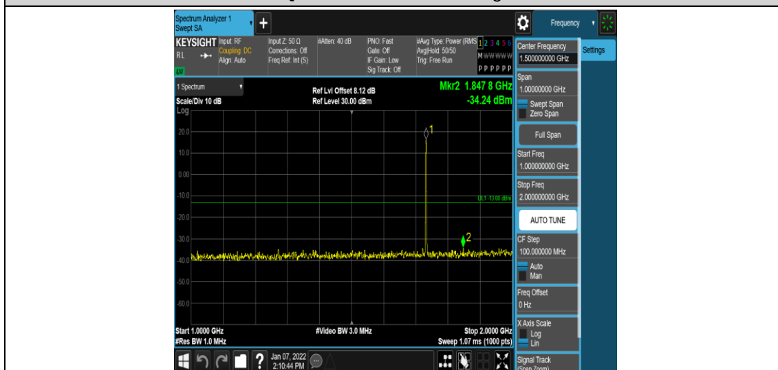
Band4-1.4MHz-QPSK-20175-1RB#0-Range4:1000~2000MHz
