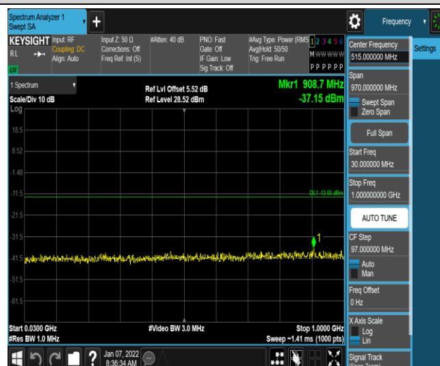
Band2-3MHz-QPSK-18615-1RB#0-Range3:30~1000MHz
