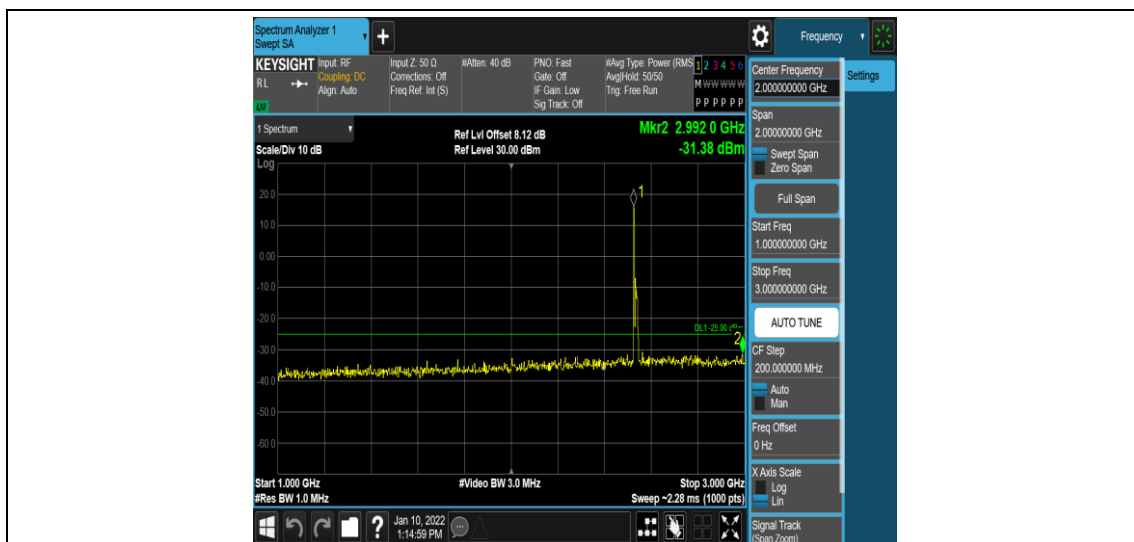
Band7-20MHz-QPSK-21100-1RB#0-Range4:1000~3000MHz
