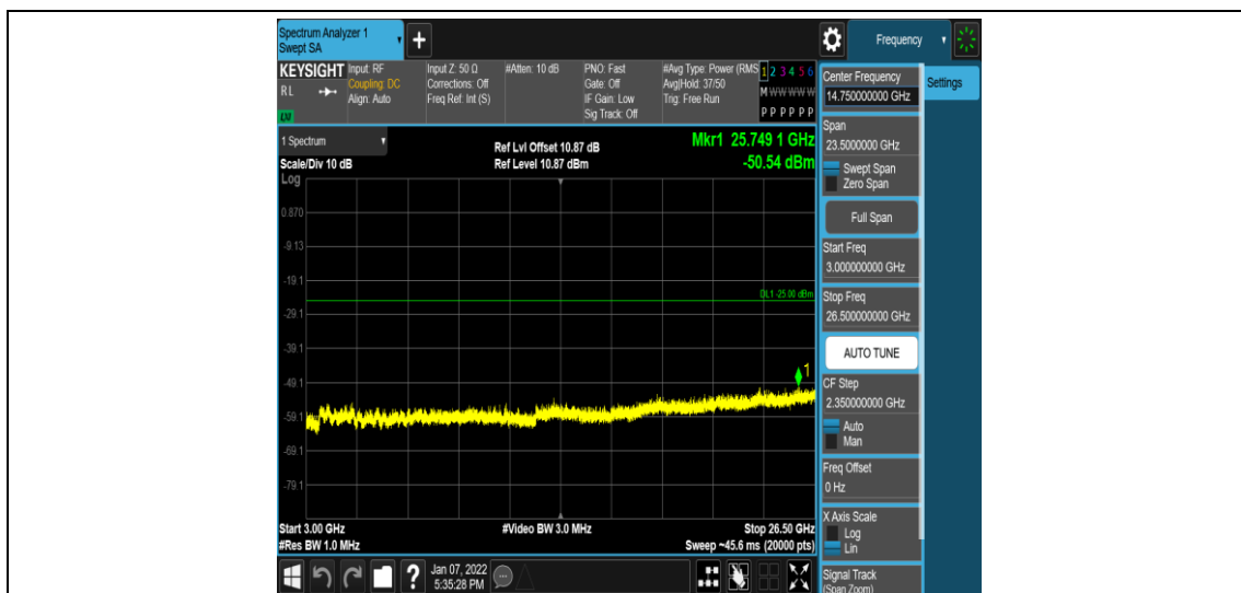
Band7-5MHz-QPSK-21425-1RB#0-Range5:3000~26500MHz
