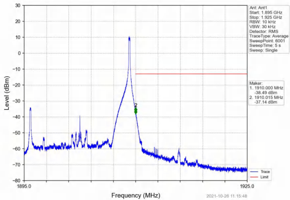
Band2_15MHz_QPSK_HCH_1902.5MHz_RB_1_74_NTNV
