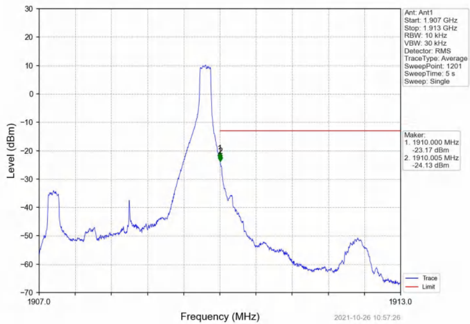
Band2_3MHz_QPSK_HCH_1908.5MHz_RB_1_14_NTNV
