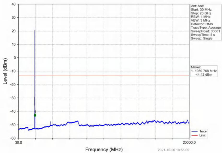
Band2_3MHz_QPSK_MCH_1880MHz_RB_1_0_NTNV
