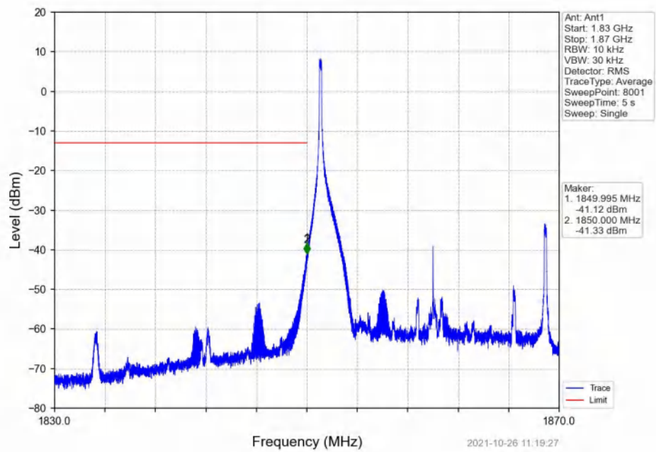
Band2_20MHz_16QAM_LCH_1860MHz_RB_1_0_NTNV
