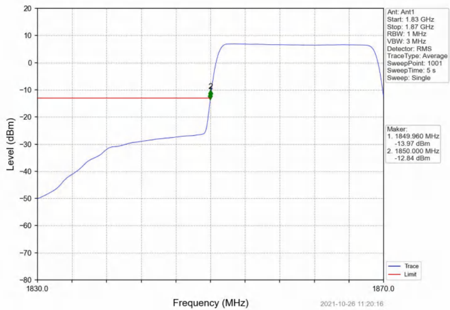
Band2_20MHz_16QAM_LCH_1860MHz_RB_100_0_NTNV
