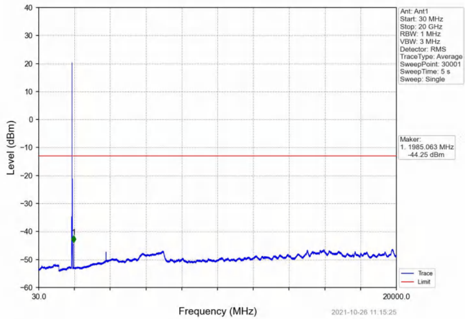
Band2_15MHz_QPSK_HCH_1902.5MHz_RB_1_74_NTNV
