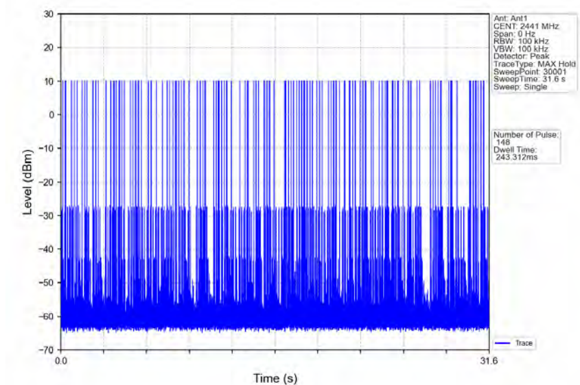
GFSK_DH3_HOPP_Ant1_NTNV
