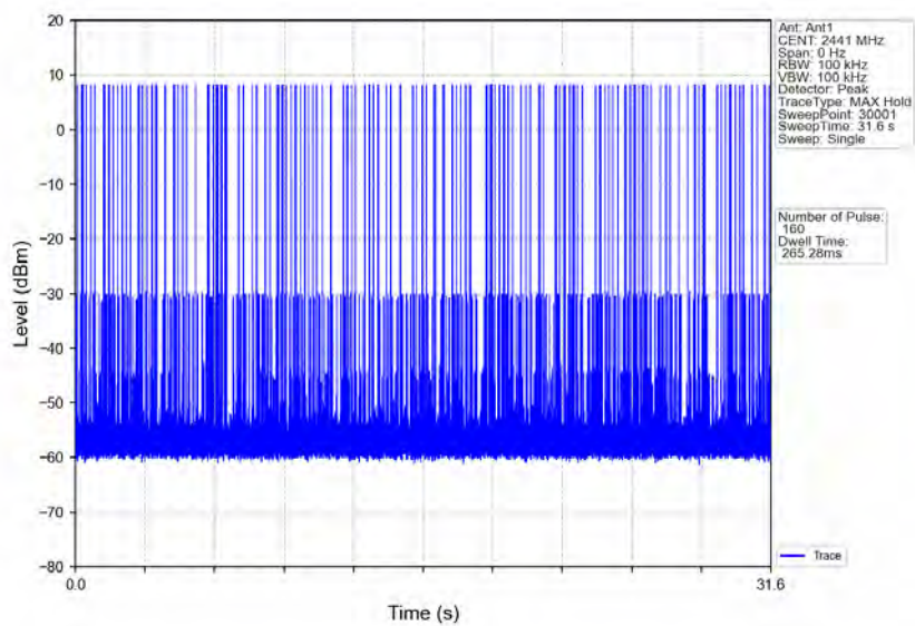
Pi/4DQPSK_2DH3_HOPP_Ant1_NTNV
