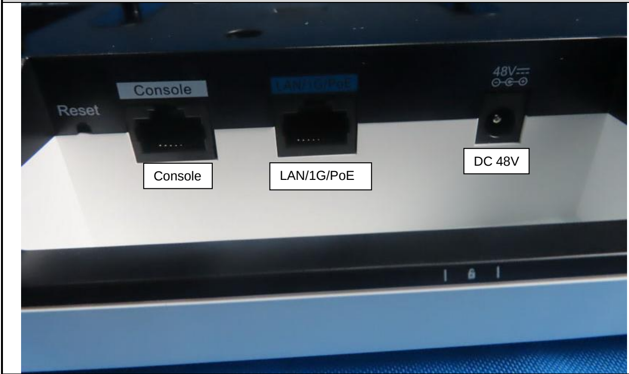
EUT Photo
