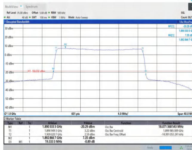
Band2-20MHz-16QAM-18700-100RB#0
