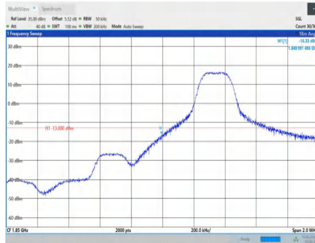
Band2-5MHz-QPSK-18625-1RB#24
