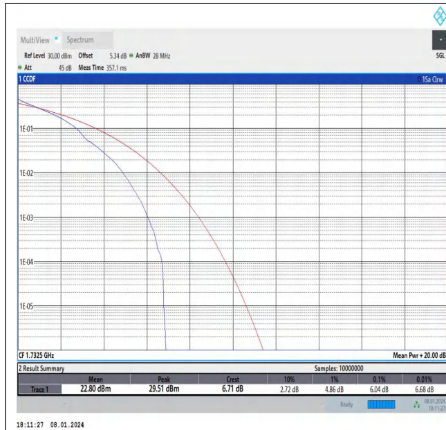
Band4-20MHz-QPSK-20175-1RB#0-PASS
