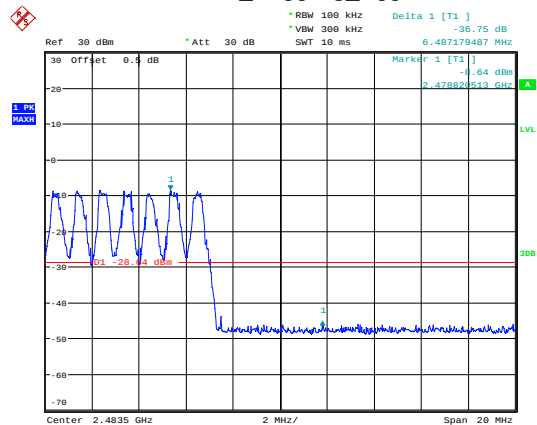
DH1_Hopping_Upper
