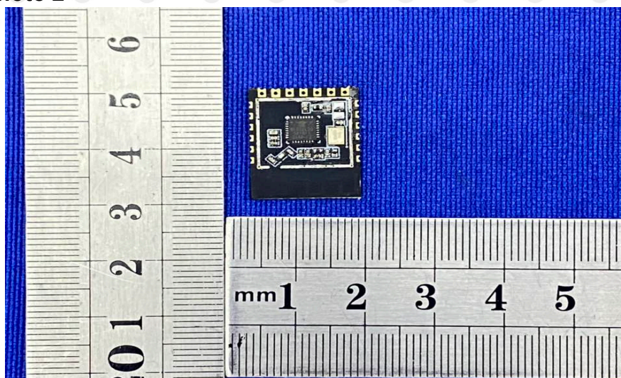
EUT Photo 2
