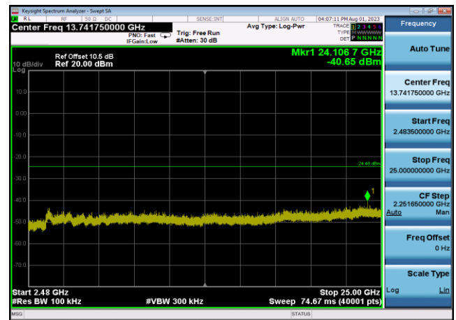
,Plot 4,2483.5MHz~25000MHz-802.11n(HT 20),2462MHz,Ant0
