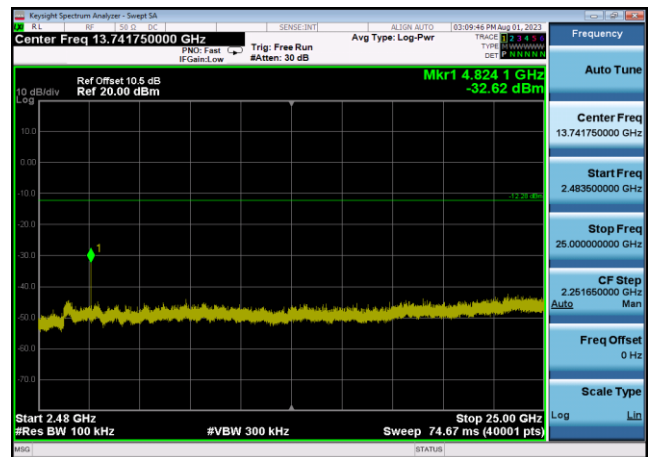
,Plot 4,2483.5MHz~25000MHz-802.11b
