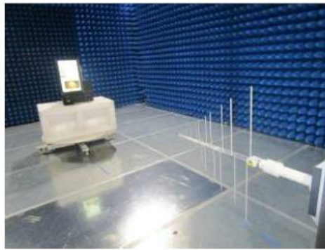
Vertical Polarisation 200MHz - 1000MHz
