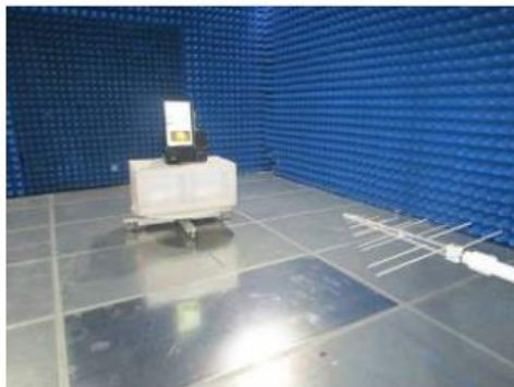
Horizontal Polarisation 200MHz - 1000MHz
