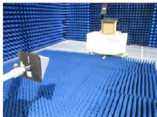
Vertical Polarisation 1000MHz - 6000MHz
