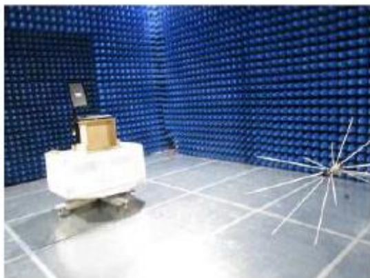
Horizontal Polarisation 30MHz - 200MHz
