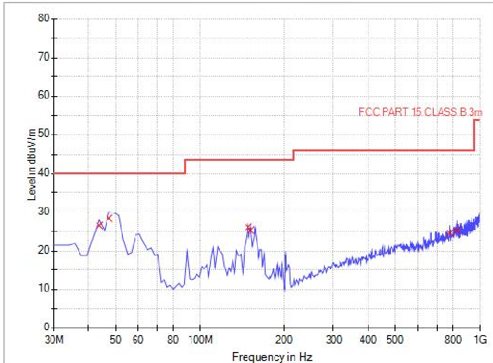
EMISweep-3M(30-1G)
