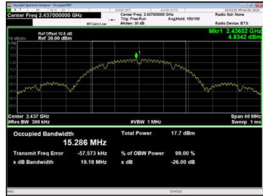
11B-Ant1-2437
