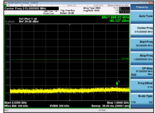
11G-Ant1-2437-30~1000-PASS
