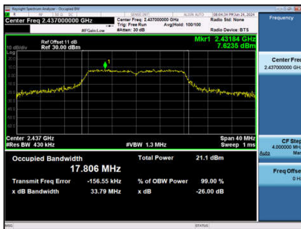
11G-Ant1-2437
