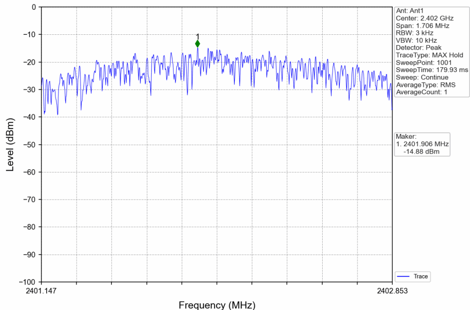
2M_LCH_2402MHz_DataRate=_Ant1_NTNV
