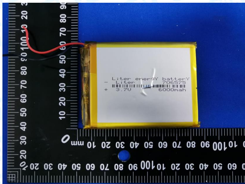
Photo 6 Battery parameters
