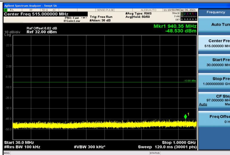
Band25-20MHz-64QAM-26365-1RB#0-30~1000MHz
