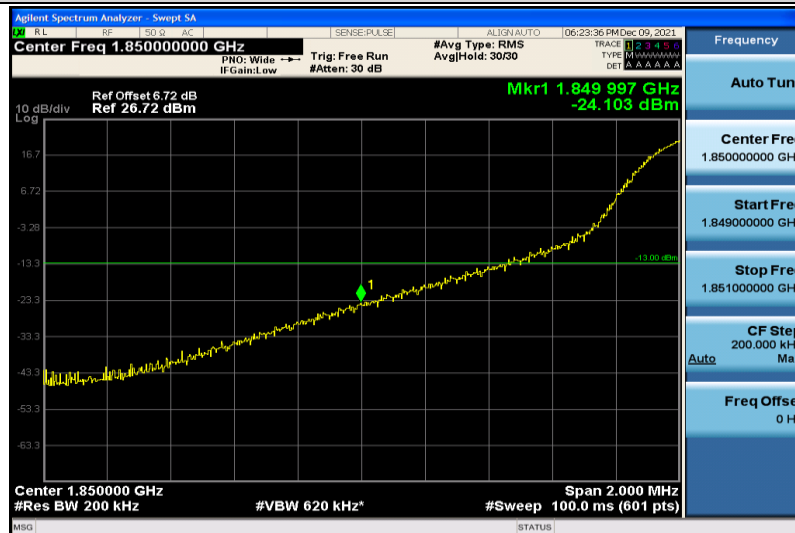
Band2-20MHz-64QAM-18700-1RB#0
