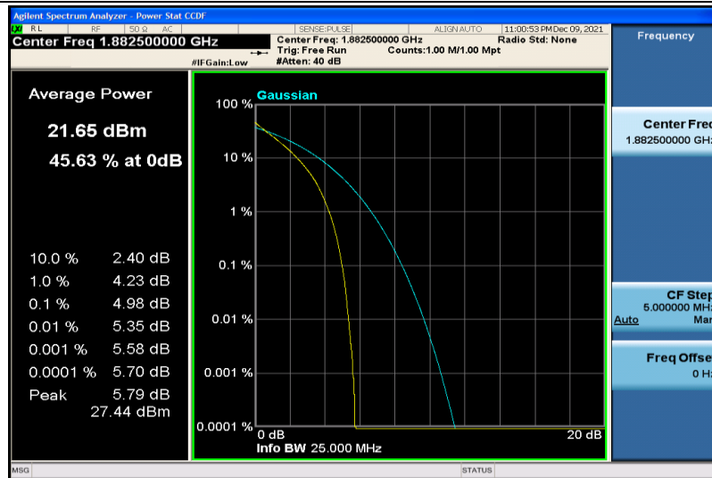
Band25-10MHz-64QAM-26365-50RB#0
