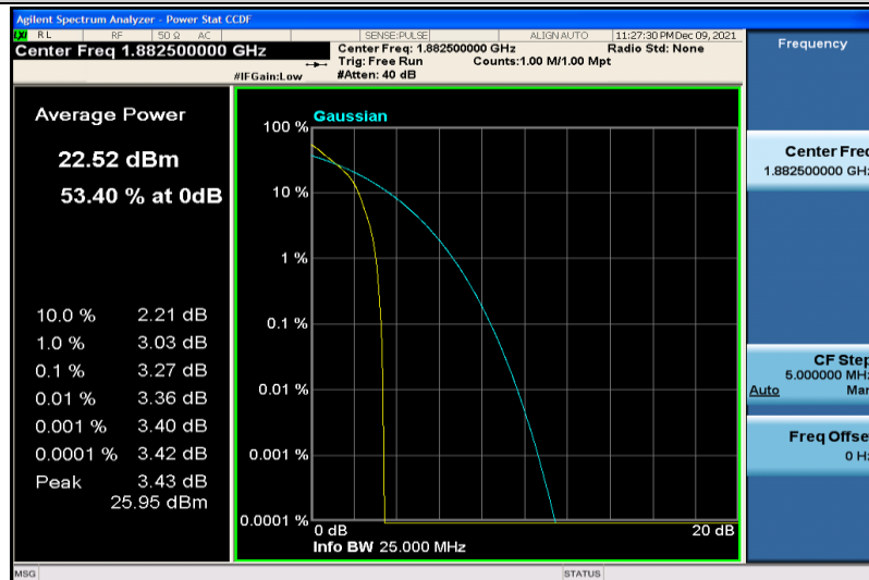
Band25-20MHz-64QAM-26365-1RB#0
