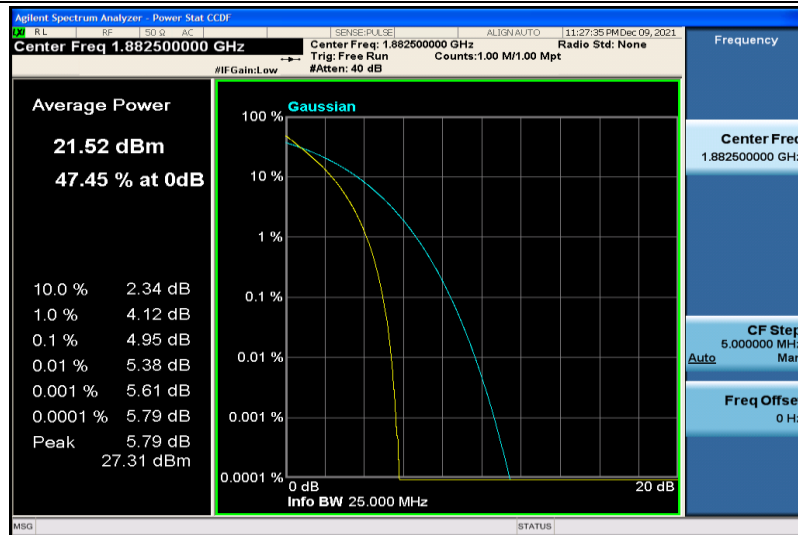
Band25-20MHz-64QAM-26365-100RB#0
