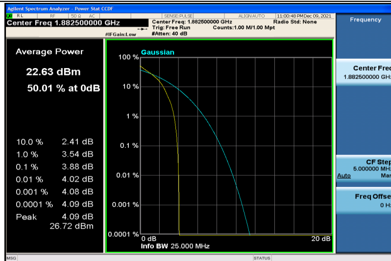
Band25-10MHz-64QAM-26365-1RB#0
