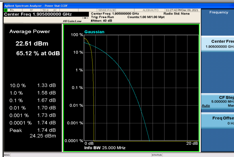
Band25-20MHz-64QAM-26590-1RB#0
