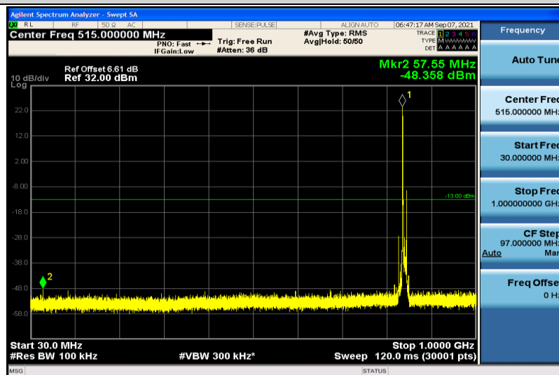
Band26-10MHz-QPSK-26990-1RB#0-30~1000MHz
