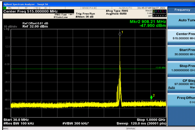
Band12-5MHz-QPSK-23155-1RB#0-30~1000MHz
