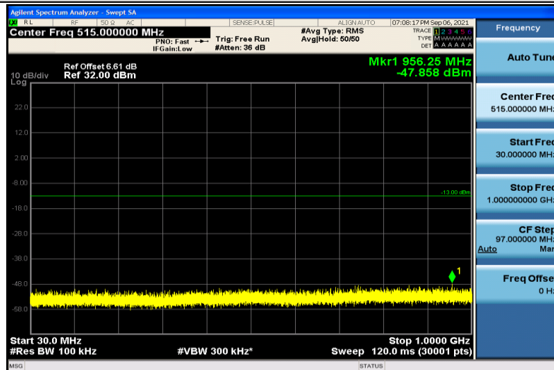
Band2-20MHz-QPSK-19100-1RB#0-30~1000MHz
