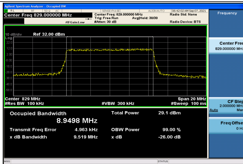
Band26-10MHz-QPSK-26840-50RB#0-8.9498
