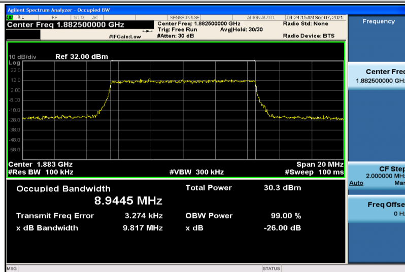
Band25-10MHz-QPSK-26365-50RB#0-8.9445
