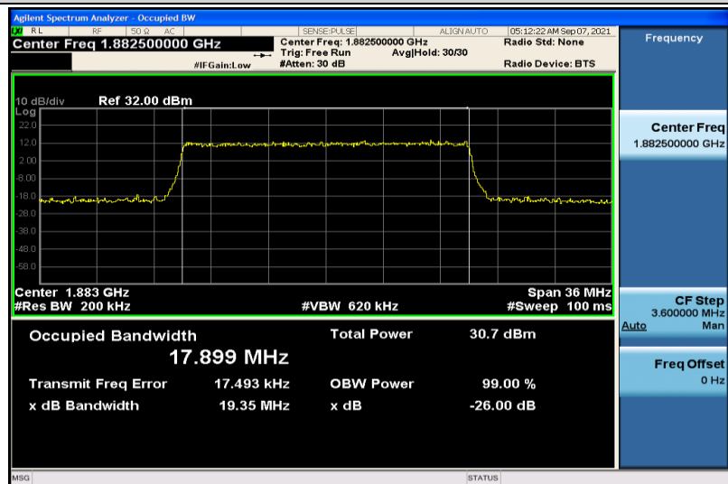
Band25-20MHz-QPSK-26365-100RB#0-17.899
