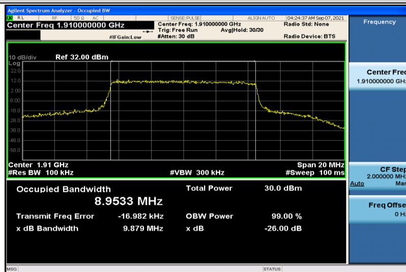
Band25-10MHz-QPSK-26640-50RB#0-8.9533
