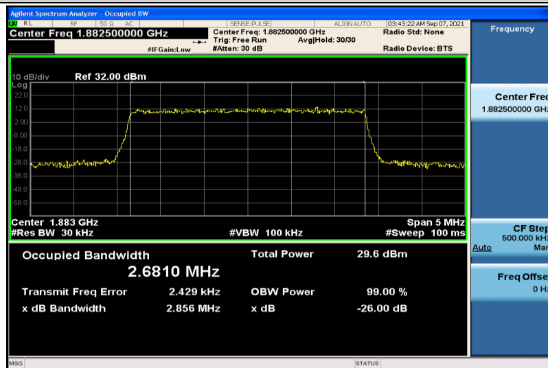
Band25-3MHz-QPSK-26365-15RB#0-2.6810
