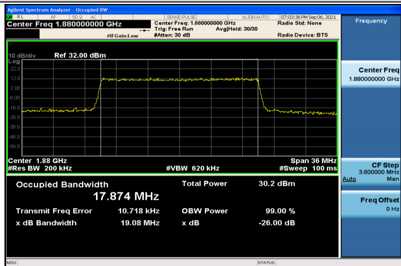
Band2-20MHz-QPSK-18900-100RB#0-17.874
