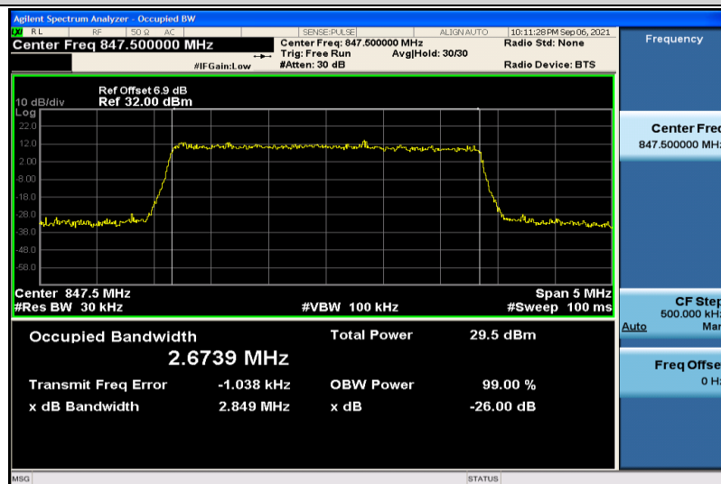
Band5-3MHz-QPSK-20635-15RB#0-2.6739
