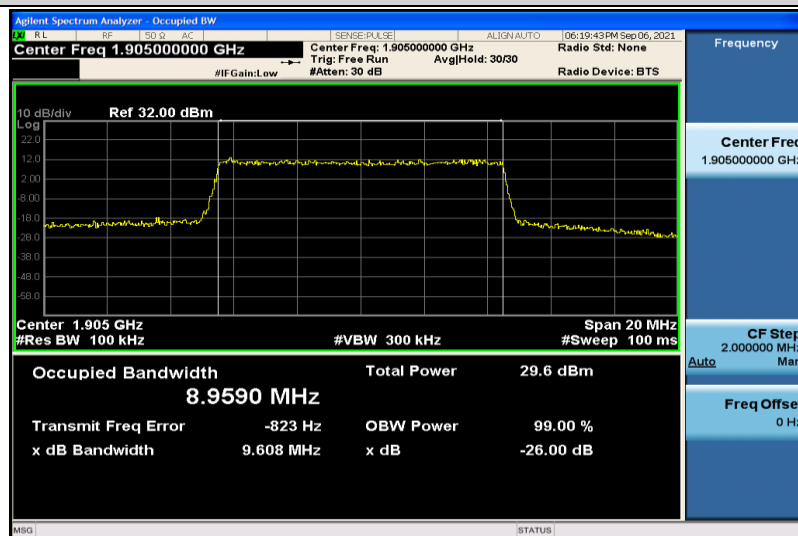
Band2-10MHz-QPSK-19150-50RB#0-8.9590
