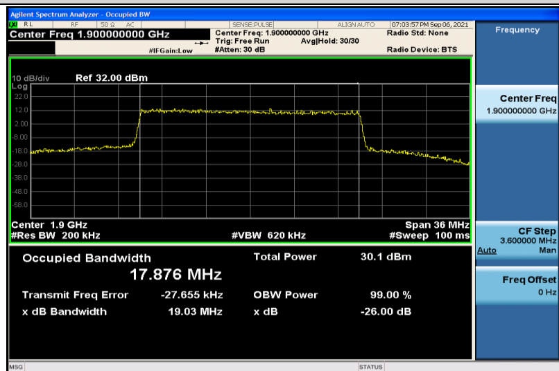
Band2-20MHz-QPSK-19100-100RB#0-17.876
