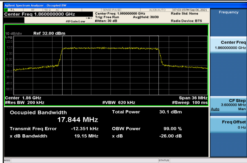
Band2-20MHz-QPSK-18700-100RB#0-17.844
