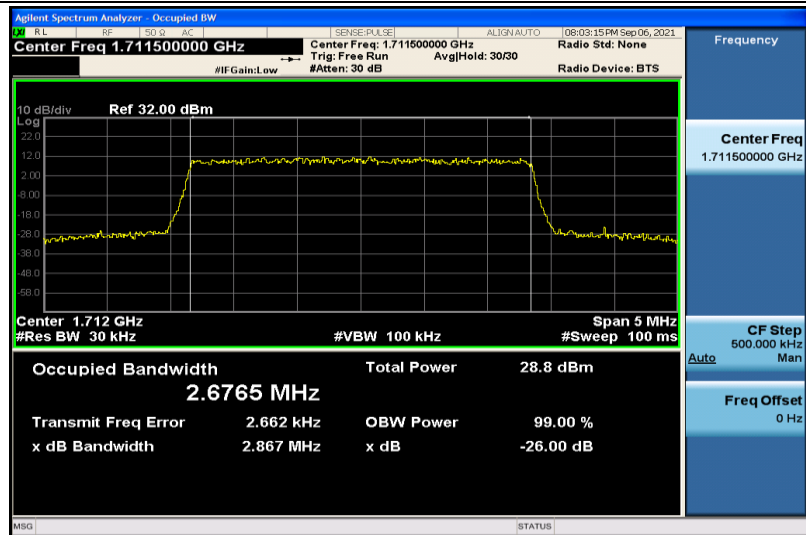
Band4-3MHz-QPSK-19965-15RB#0-2.6765
