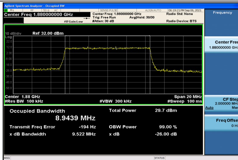
Band2-10MHz-QPSK-18900-50RB#0-8.9439
