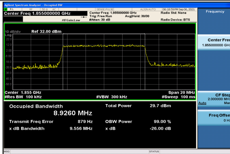
Band2-10MHz-QPSK-18650-50RB#0-8.9260
