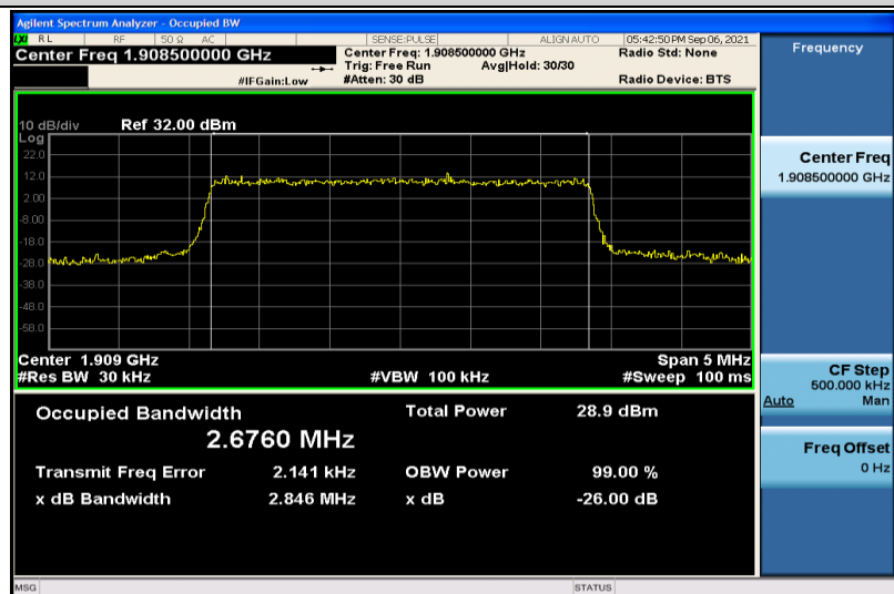
Band2-3MHz-QPSK-19185-15RB#0-2.6760
