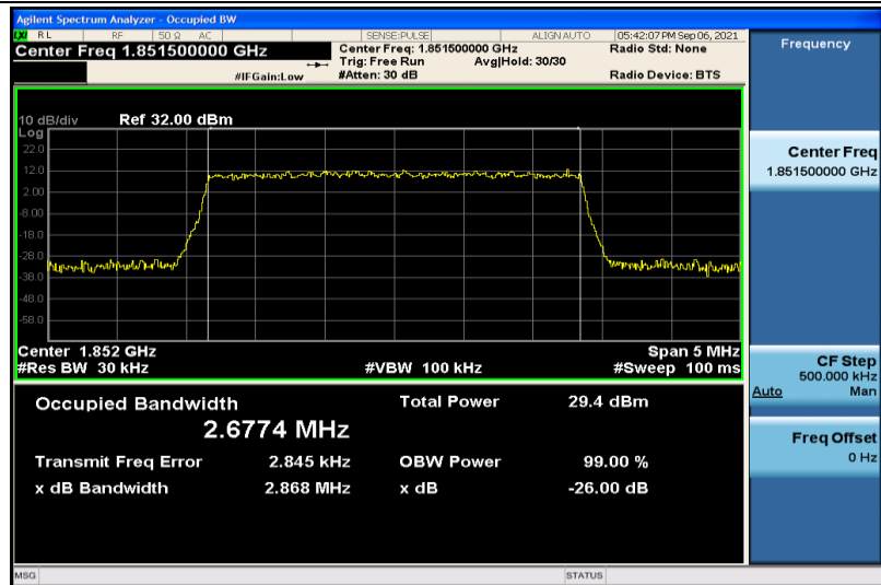
Band2-3MHz-QPSK-18615-15RB#0-2.6774
