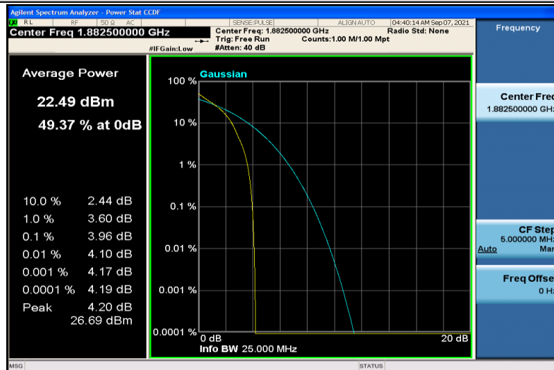
Band25-10MHz-QPSK-26365-1RB#0
