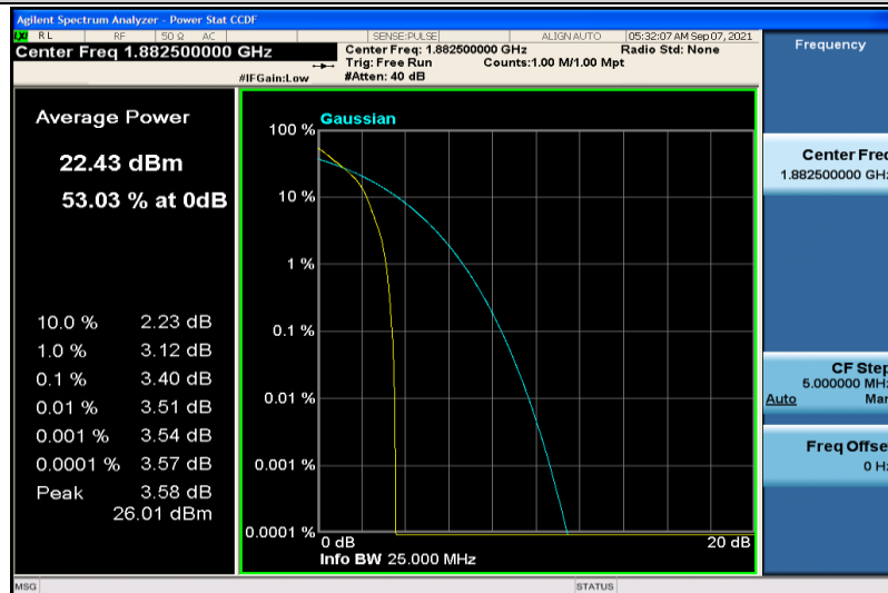
Band25-20MHz-QPSK-26365-1RB#0
