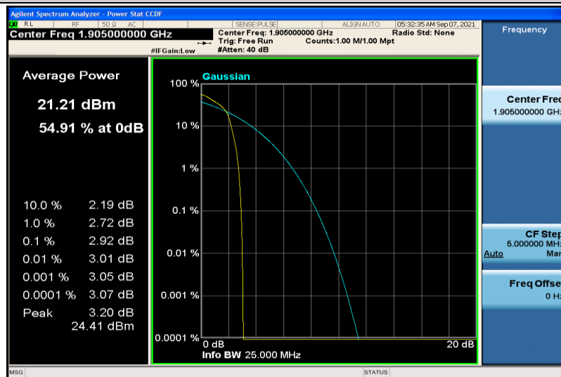
Band25-20MHz-16QAM-26590-1RB#0
