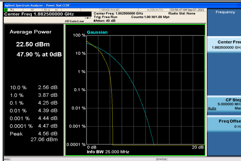
Band25-3MHz-QPSK-26365-1RB#0
