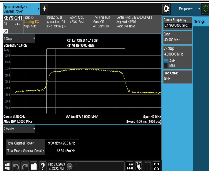
11AX20CDD_Ant1_5180
