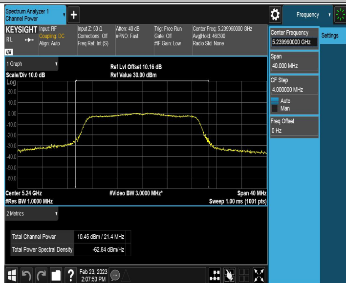
11AC20CDD_Ant1_5240
