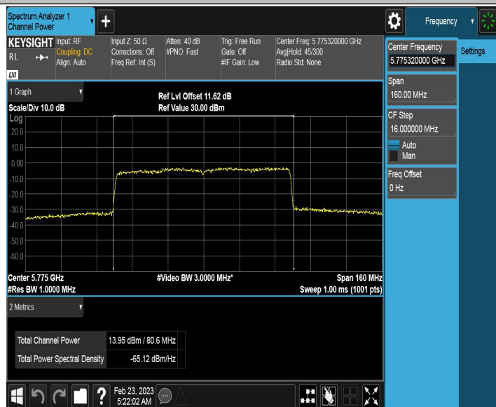
11AX80ISO_Ant2_5775
