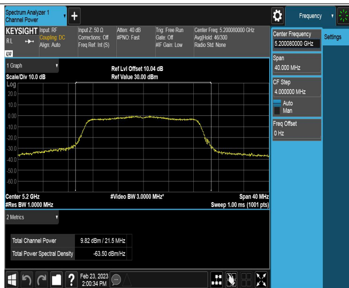
11AC20CDD_Ant2_5200
