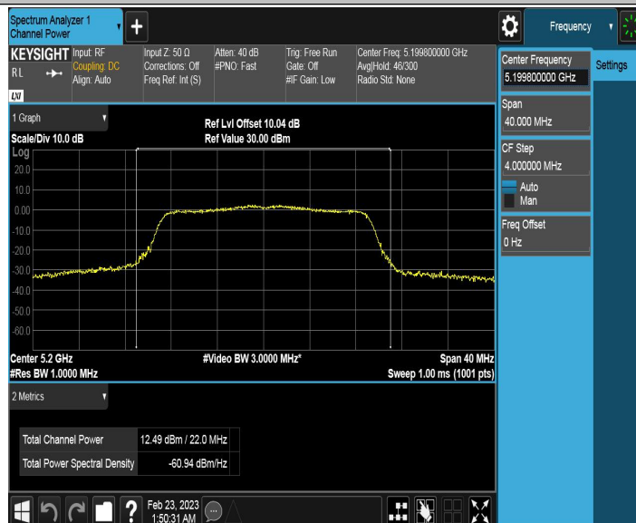
11AX20SISO_Ant2_5200
