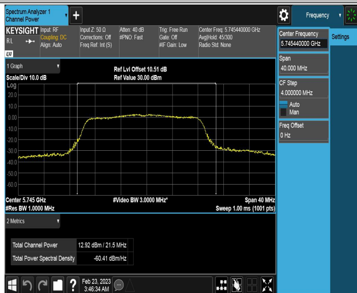
11N20SISO_Ant2_5745
