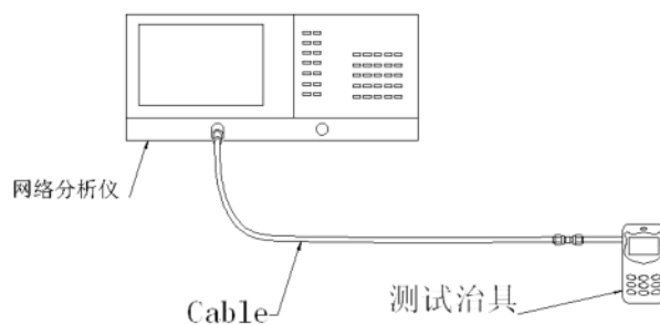
测试示意图
