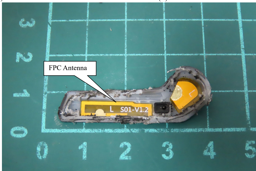
(10) EUT Photo - M/N: ROG CETRA TRUE WIRELESS(L)
