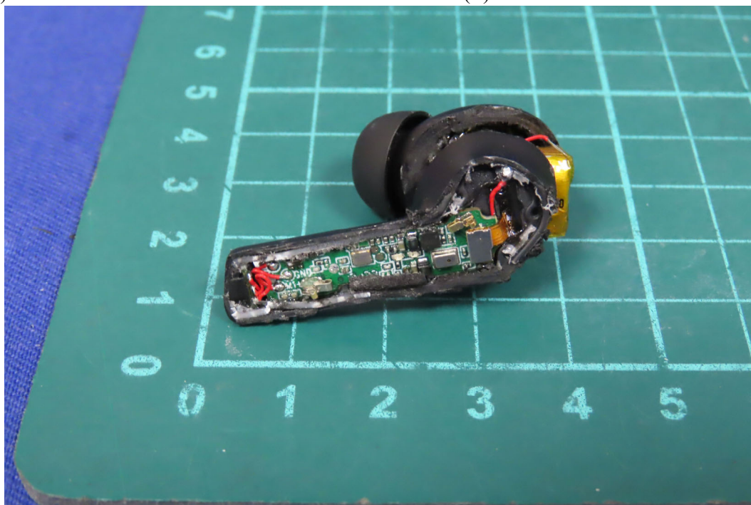
(11) EUT Photo - M/N: ROG CETRA TRUE WIRELESS(L)
