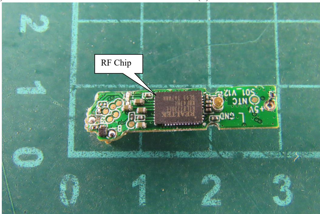
(14) EUT Photo - M/N: ROG CETRA TRUE WIRELESS(L)
