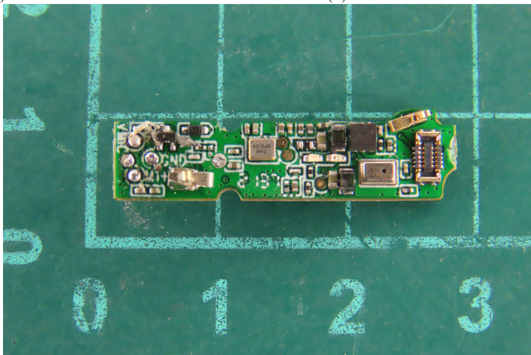
(13) EUT Photo - M/N: ROG CETRA TRUE WIRELESS(L)
