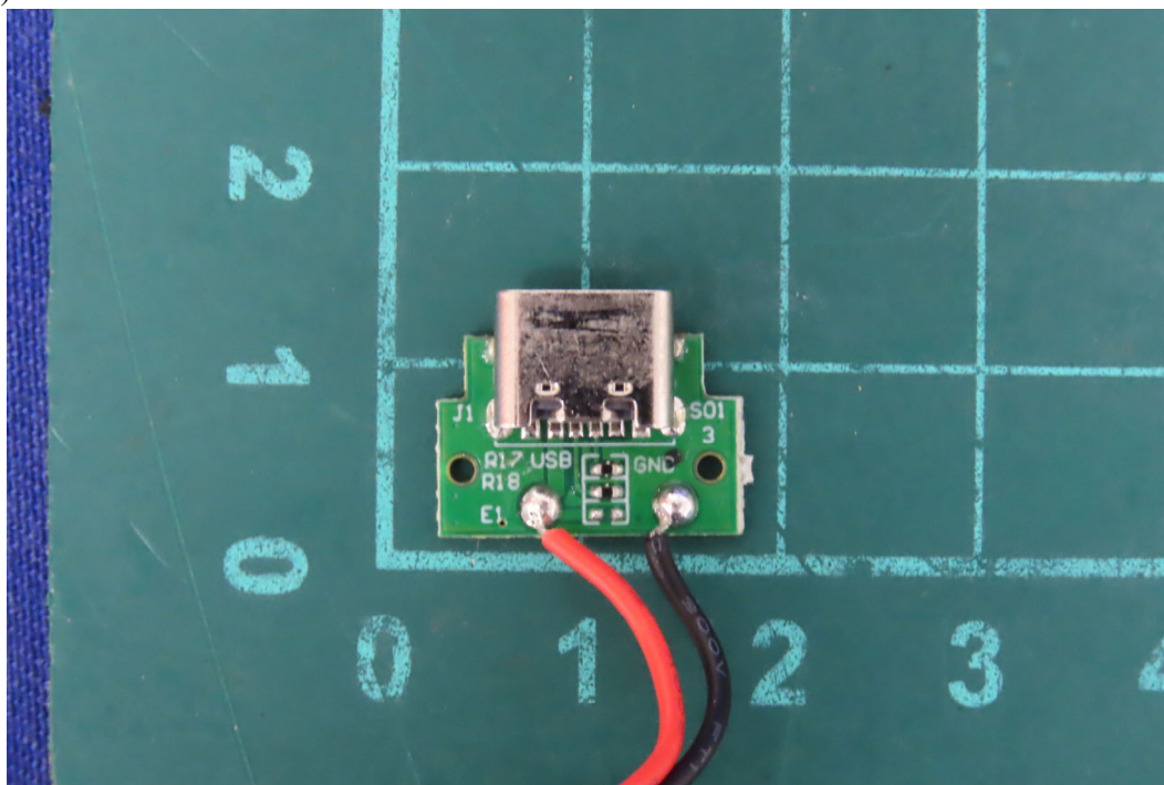
(19) EUT Photo
