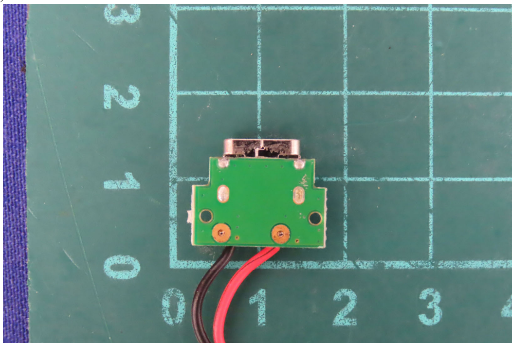
(20) EUT Photo
