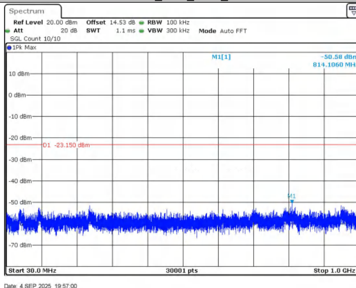
\pi /4DQPSK_Ant1_2480_30~1000
