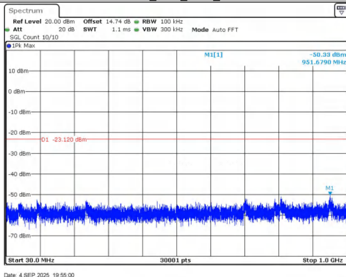
\pi /4DQPSK_Ant1_2402_30~1000
