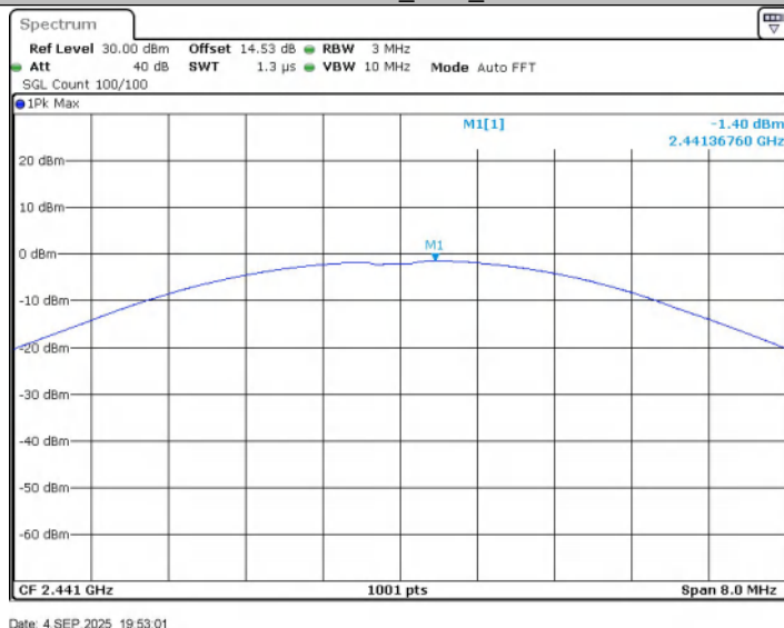
\pi /4DQPSK_Ant1_2441
