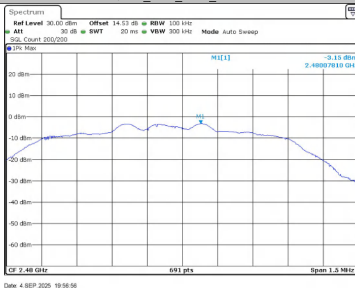
\pi /4DQPSK_Ant1_2480_0~Reference
