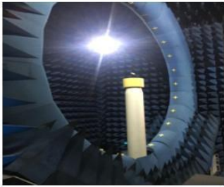
SATIMO 暗室
