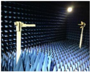
ETS 暗室
