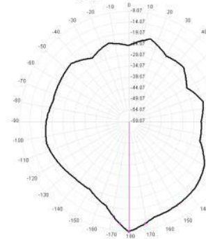
2400.0MHz Total(E1), Max=-9.07dBi
