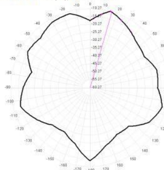
5750.0MHz Total(E1), Max=-10.27dBi
