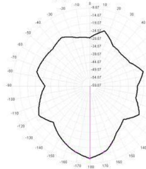
2400.0MHz Total(E2), Max=-12.57dBi
