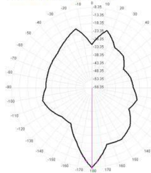
2450.0MHz Total(E1), Max=-8.35dBi
