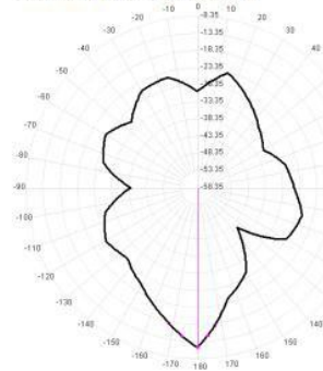
2450.0MHz Total(E2), Max=-11.88dBi
