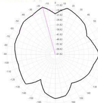
5850.0MHz Total(E1), Max=-11.82dBi
