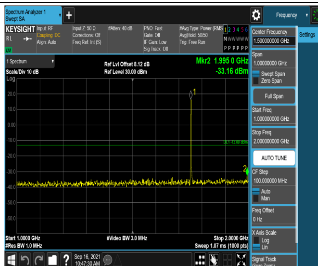
Band4-3MHz-QPSK-20385-1RB#0-Range4:1000~2000MHz
