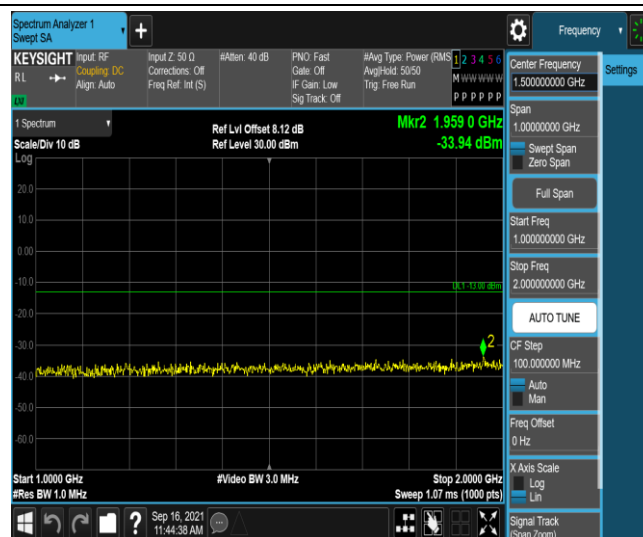
Band4-5MHz-QPSK-20375-1RB#0-Range4:1000~2000MHz
