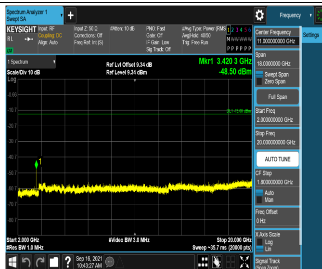
Band4-3MHz-QPSK-19965-1RB#0-Range5:2000~20000MHz
