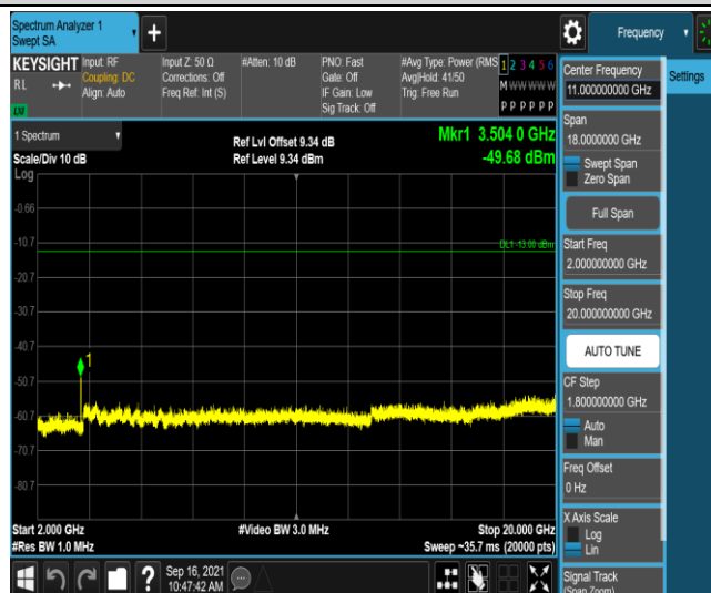
Band4-3MHz-QPSK-20385-1RB#0-Range5:2000~20000MHz
