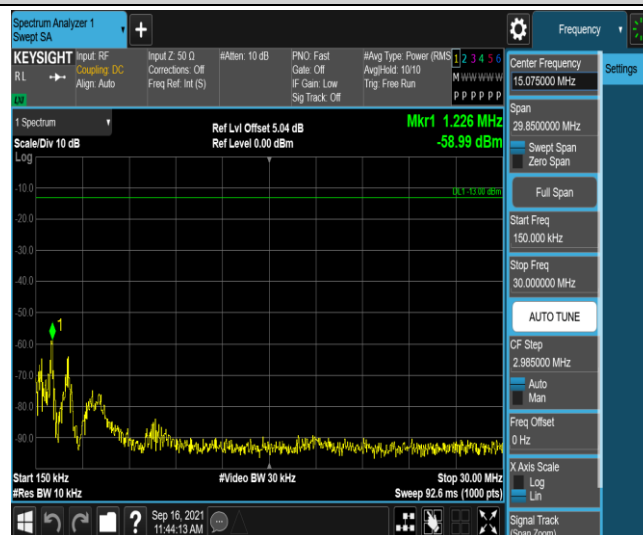
Band4-5MHz-QPSK-20375-1RB#0-Range2:0.15~30MHz
