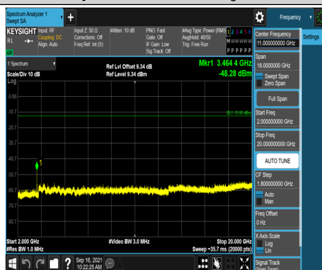
Band4-1.4MHz-QPSK-20175-1RB#0-Range5:2000~20000MHz
