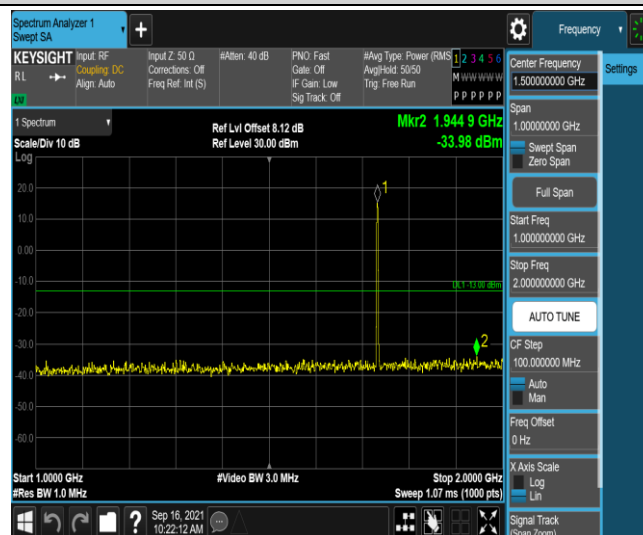
Band4-1.4MHz-QPSK-20175-1RB#0-Range4:1000~2000MHz
