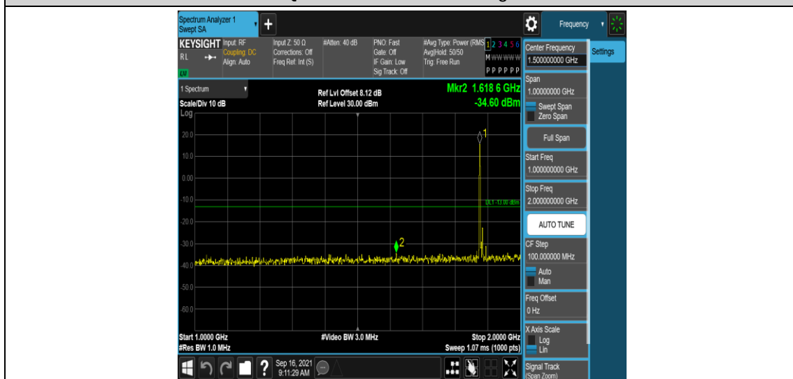
Band2-10MHz-QPSK-18900-1RB#0-Range4:1000~2000MHz
