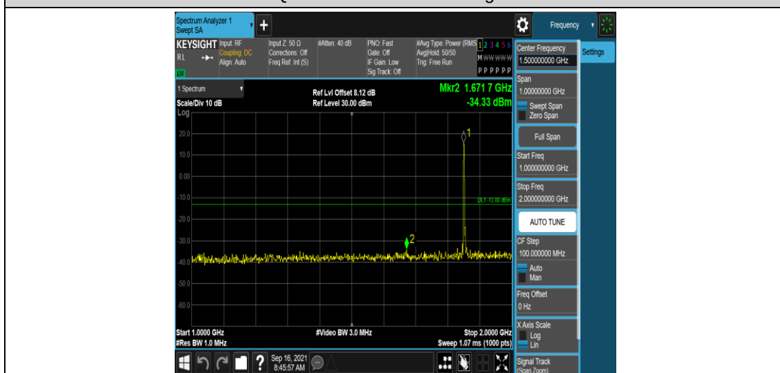
Band2-5MHz-QPSK-18625-1RB#0-Range4:1000~2000MHz
