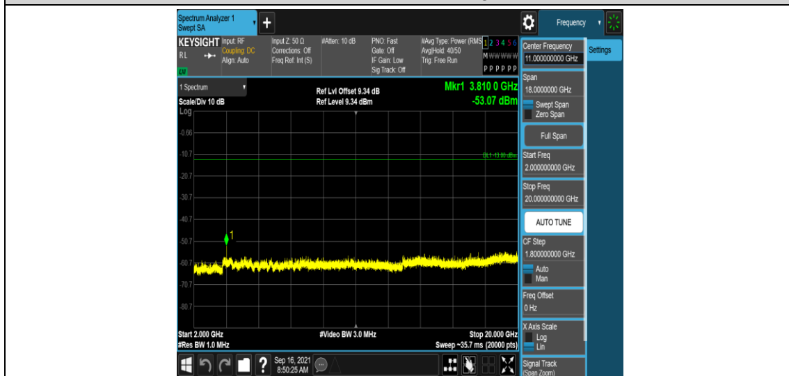
Band2-5MHz-QPSK-19175-1RB#0-Range5:2000~20000MHz
