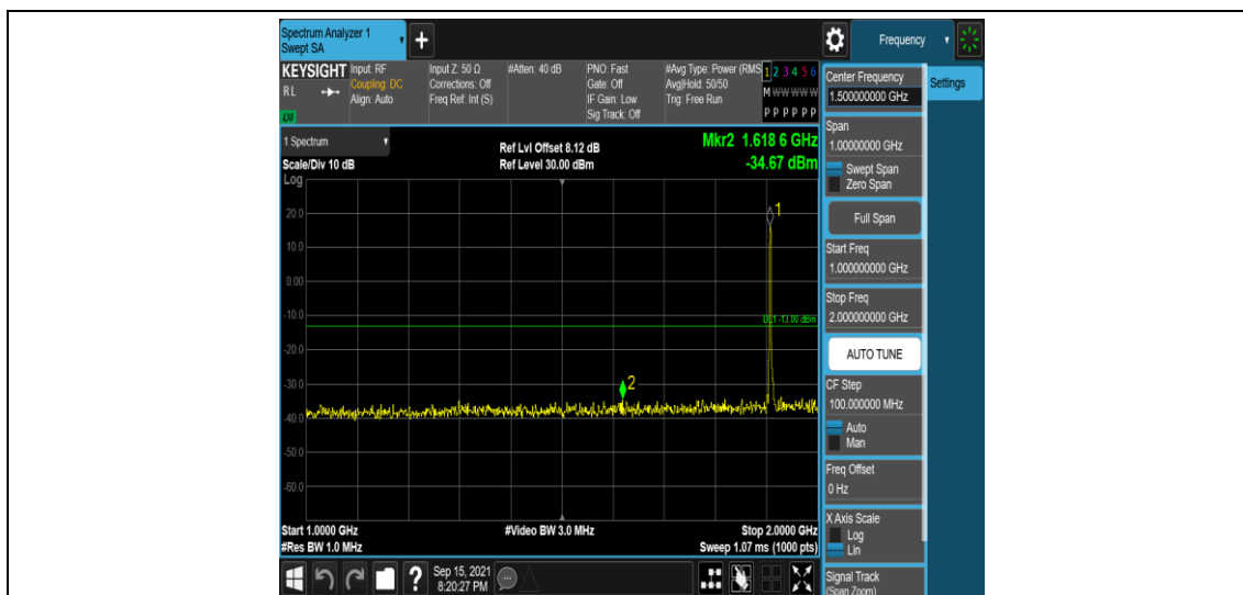
Band2-3MHz-QPSK-19185-1RB#0-Range4:1000~2000MHz
