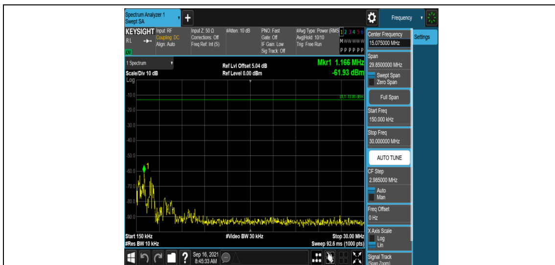
Band2-5MHz-QPSK-18625-1RB#0-Range2:0.15~30MHz
