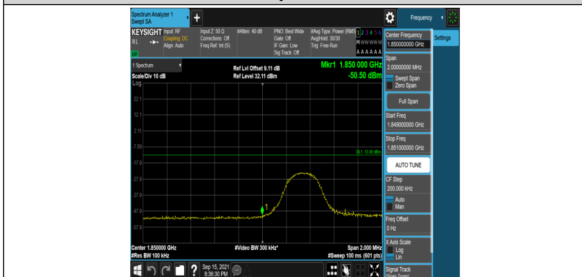
Band2-5MHz-QPSK-18625-1RB#24
