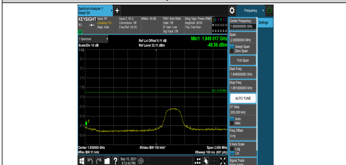
Band2-3MHz-QPSK-18615-1RB#14
