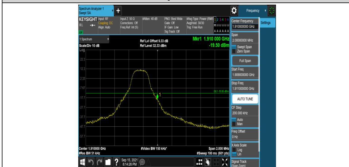
Band2-3MHz-QPSK-19185-1RB#14
