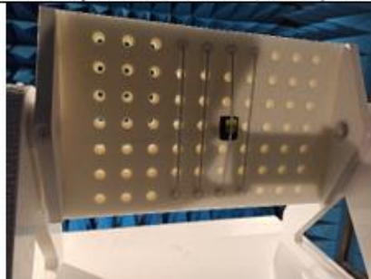
Photo Setup : anechoic chamber (Z axis)
