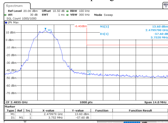
BLE 2Mbps High
