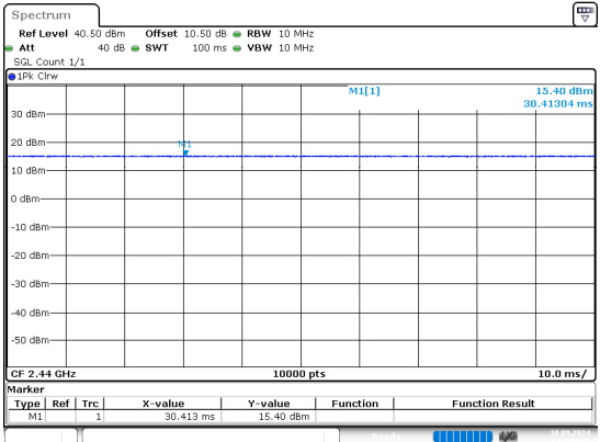
BLE 2Mbps Middle
