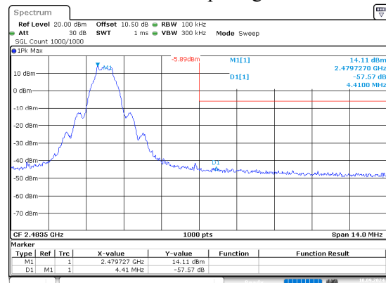
BLE 1Mbps High
