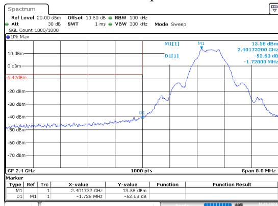
BLE 1Mbps Low
