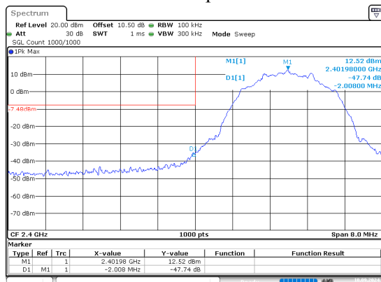
BLE 2Mbps Low
