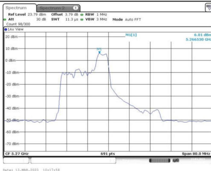
11AX40MIMO_Ant1_5270 52/40
