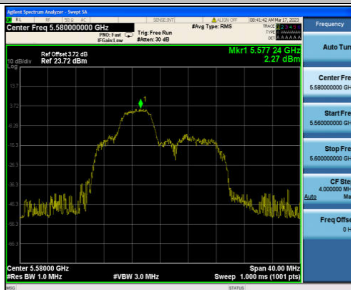
11AX20MIMO_Ant2_5580 52/38
