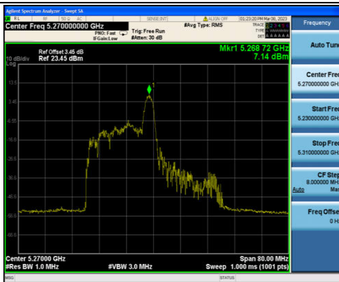
11AX40MIMO_Ant2_5270 26/8
