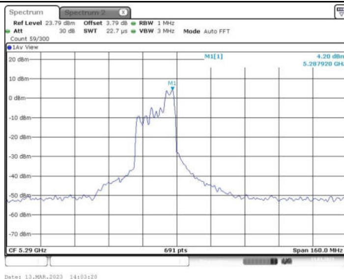
11AX80MIMO_Ant1_5290 106/56
