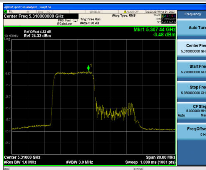
11AX40MIMO_Ant2_5310 242/61
