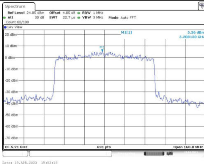
11AX80MIMO_Ant2_5210 996/67
