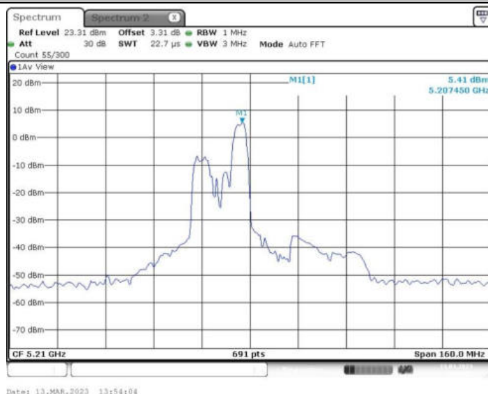
11AX80MIMO_Ant1_5210 106/56
