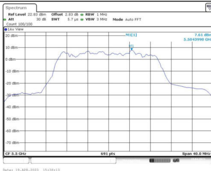
11AX20MIMO_Ant1_5500 242/61
