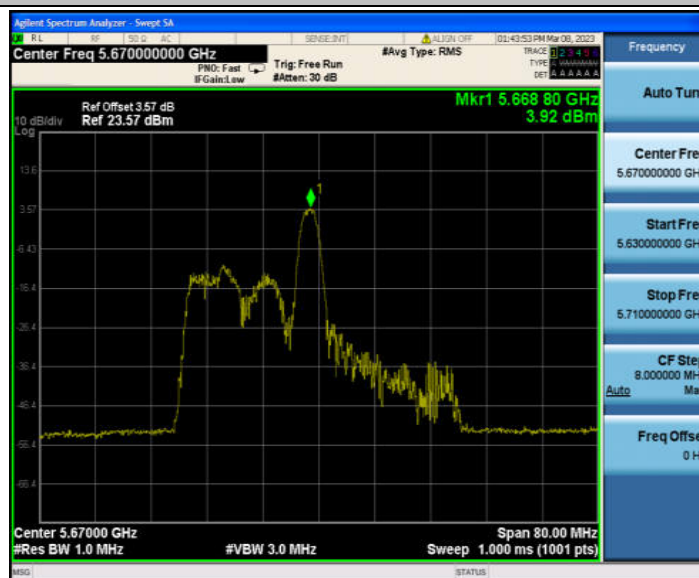
11AX40MIMO_Ant1_5670 52/40
