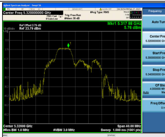
11AX20MIMO_Ant2_5320 52/38
