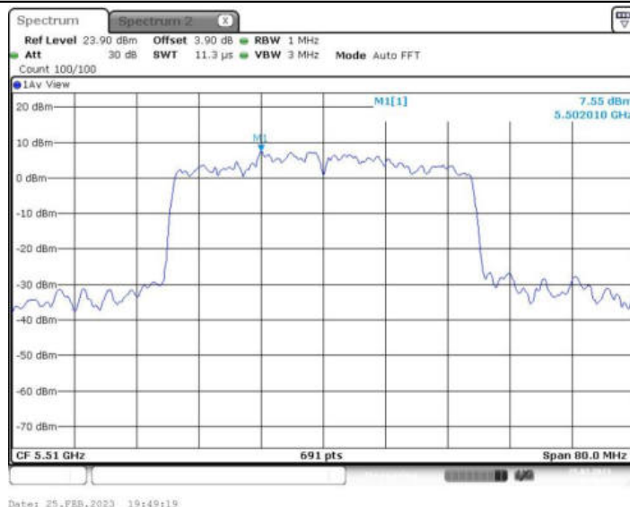
11AX40MIMO_Ant2_5510 484/65
