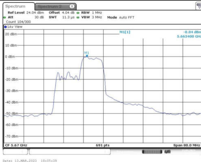
11AX40MIMO_Ant1_5670 242/61
