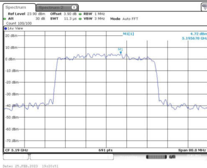
11AX40MIMO_Ant2_5190 484/65
