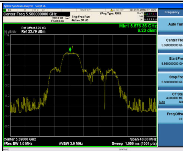
11AX20MIMO_Ant2_5580 52/38
