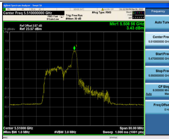
11AX40MIMO_Ant1_5510 52/40
