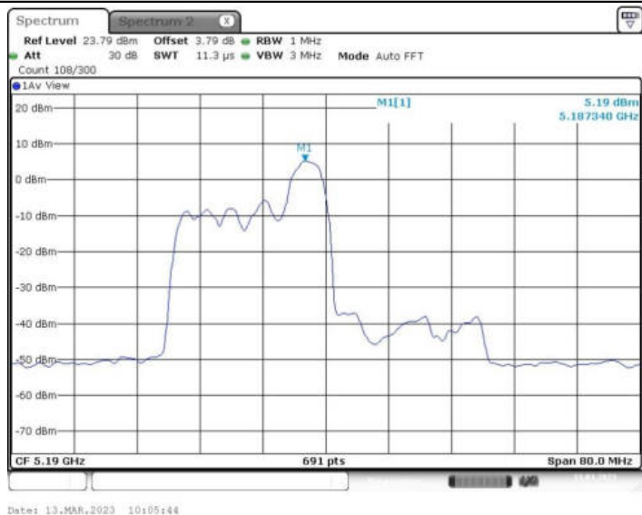
11AX40MIMO_Ant1_5190 52/40
