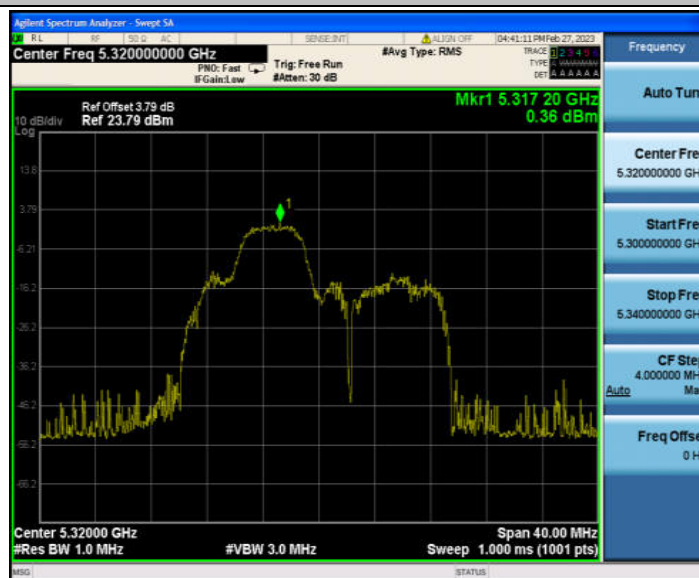
11AX20MIMO_Ant1_5320 106/53
