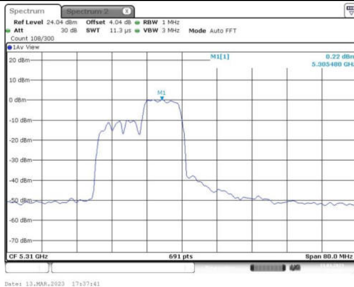
11AX40MIMO_Ant1_5310 242/61
