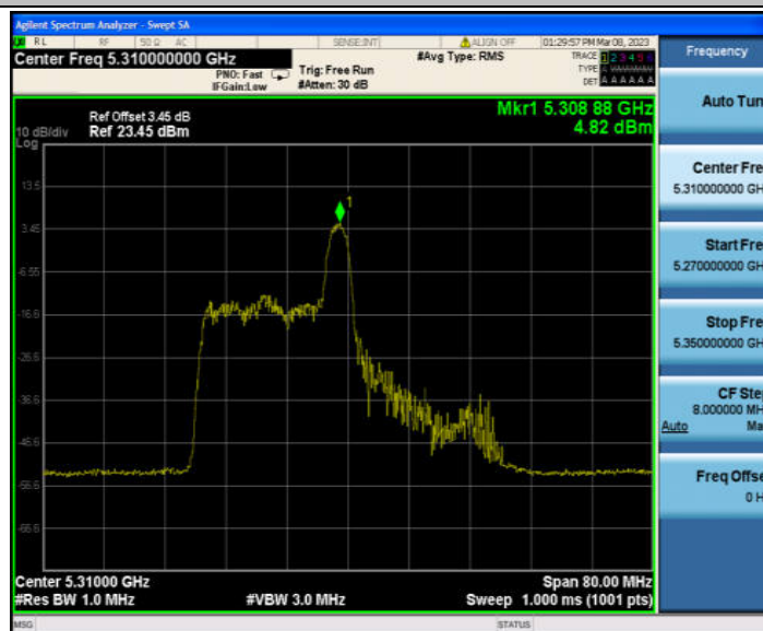
11AX40MIMO_Ant1_5310 52/40
