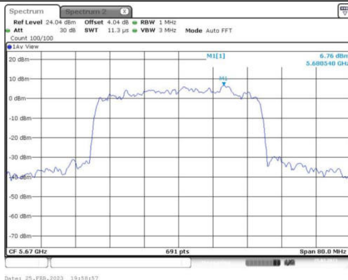
11AX40MIMO_Ant2_5670 484/65
