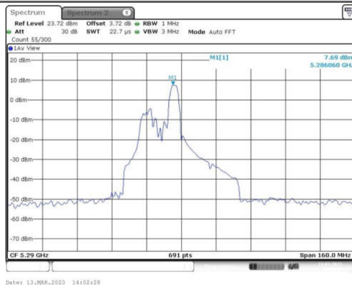
11AX80MIMO_Ant2_5290 52/44
