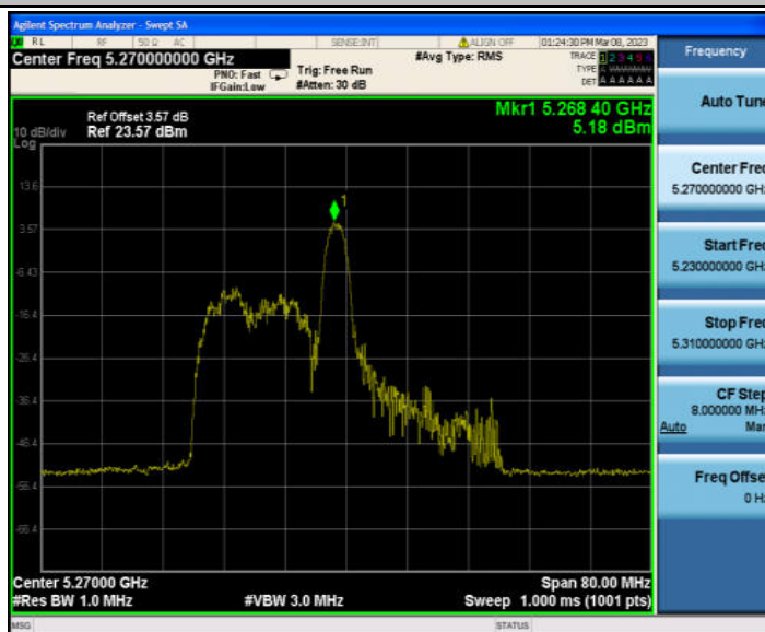
11AX40MIMO_Ant1_5270 52/40
