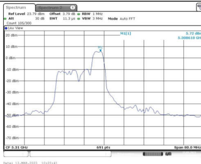
11AX40MIMO_Ant1_5310 52/40
