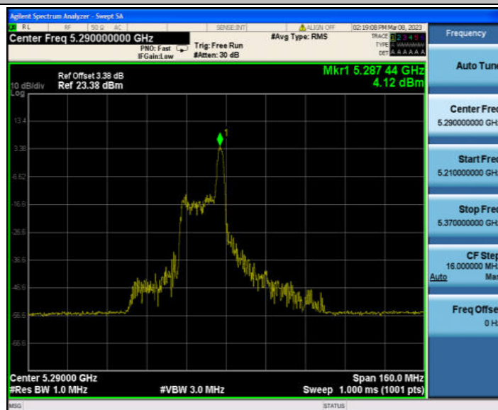
11AX80MIMO_Ant1_5290 52/44
