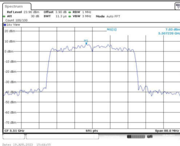
11AX40MIMO_Ant1_5510 26/8
