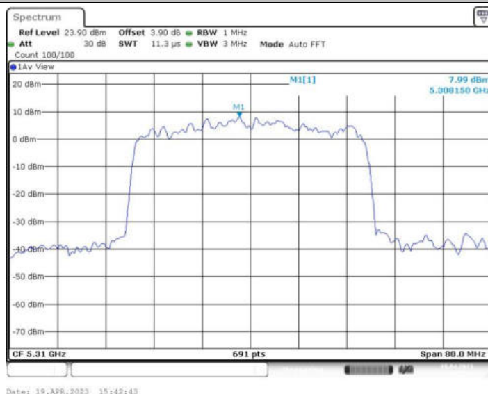
11AX40MIMO_Ant2_5310 484/65
