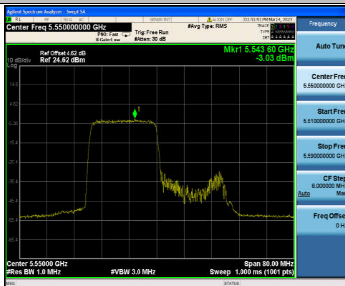
11AX40MIMO_Ant2_5550 242/61
