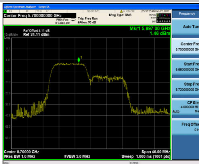
11AX20MIMO_Ant2_5700 106/53
