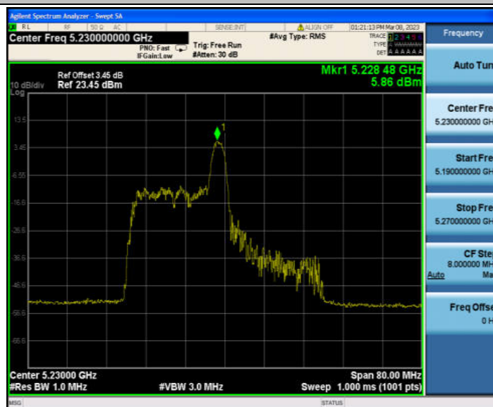
11AX40MIMO_Ant1_5230 52/40
