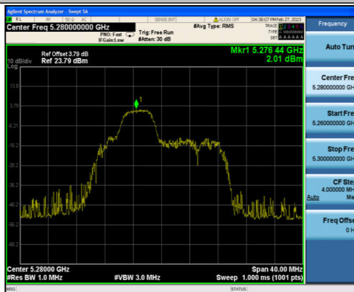
11AX20MIMO_Ant1_5280 106/53
