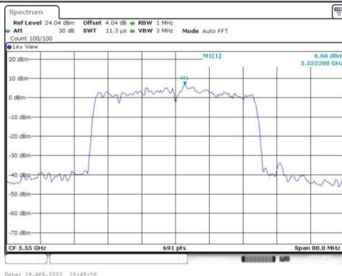
11AX40MIMO_Ant2_5550 484/65
