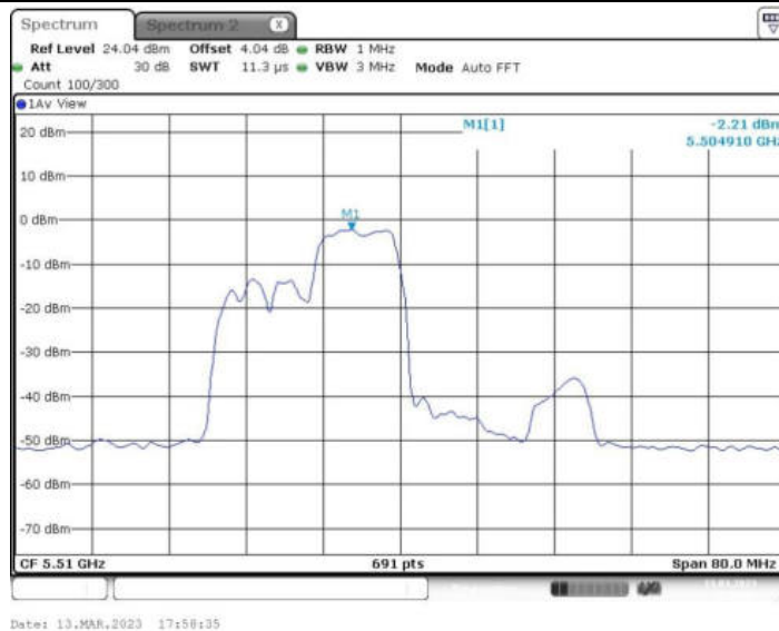
11AX40MIMO_Ant1_5510 242/61
