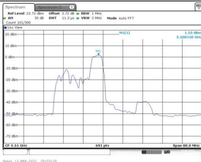
11AX40MIMO_Ant1_5510 106/54
