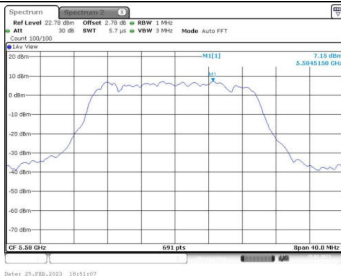
11AX20MIMO_Ant2_5580 242/61
