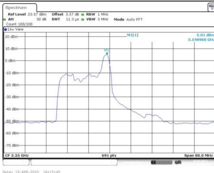
11AX40MIMO_Ant1_5550 52/40
