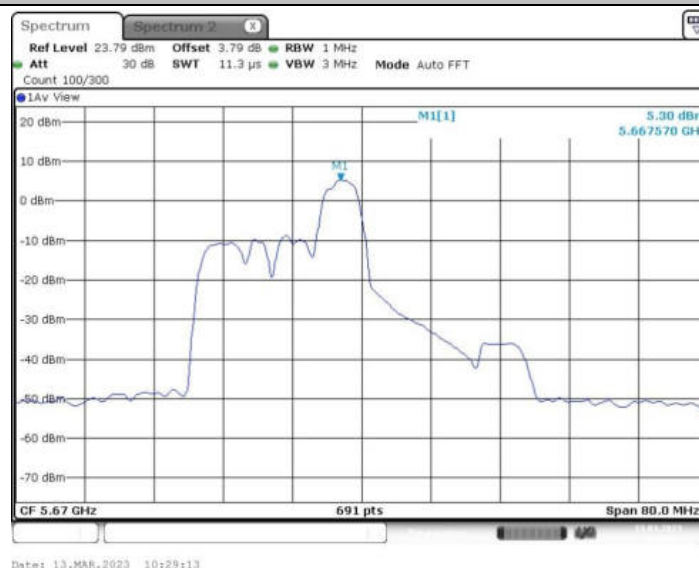
11AX40MIMO_Ant1_5670 52/40
