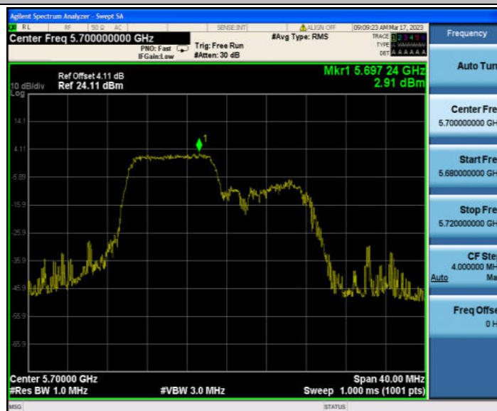
11AX20MIMO_Ant2_5700 106/53
