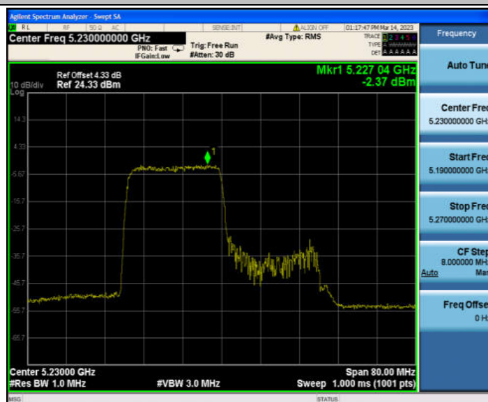
11AX40MIMO_Ant2_5230 242/61
