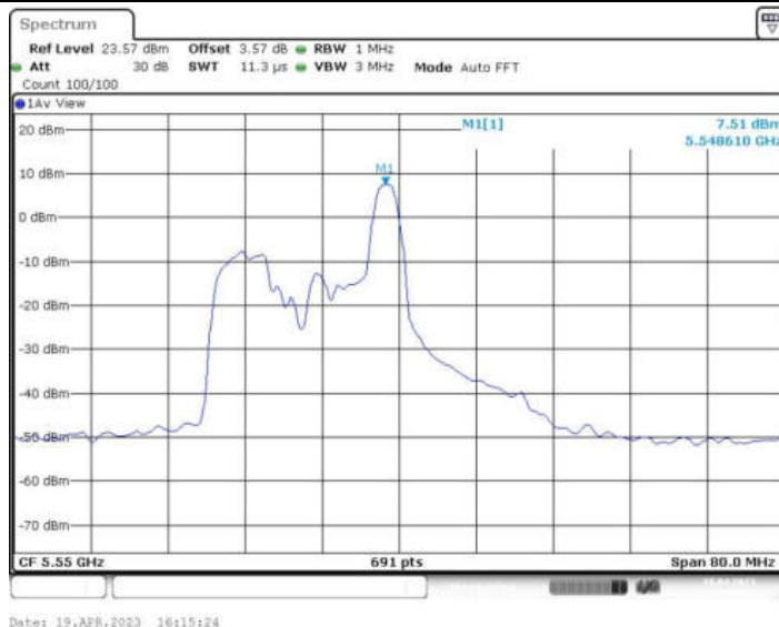
11AX40MIMO_Ant2_5550 26/8
