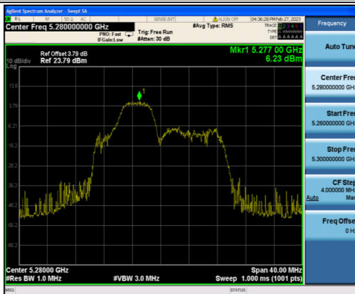
11AX20MIMO_Ant1_5280 52/38
