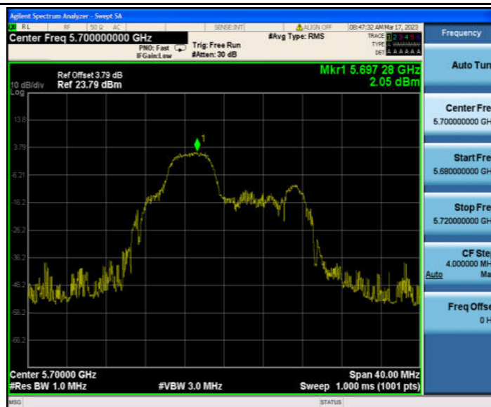
11AX20MIMO_Ant1_5700 106/53
