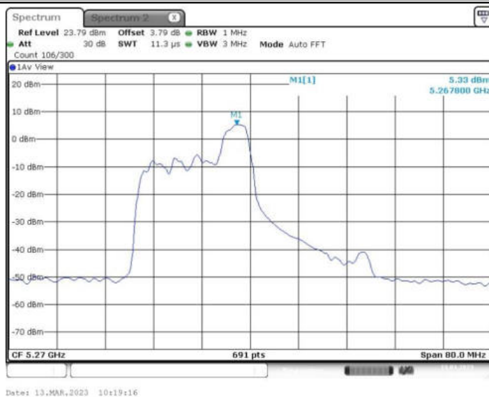
11AX40MIMO_Ant1_5270 106/54
