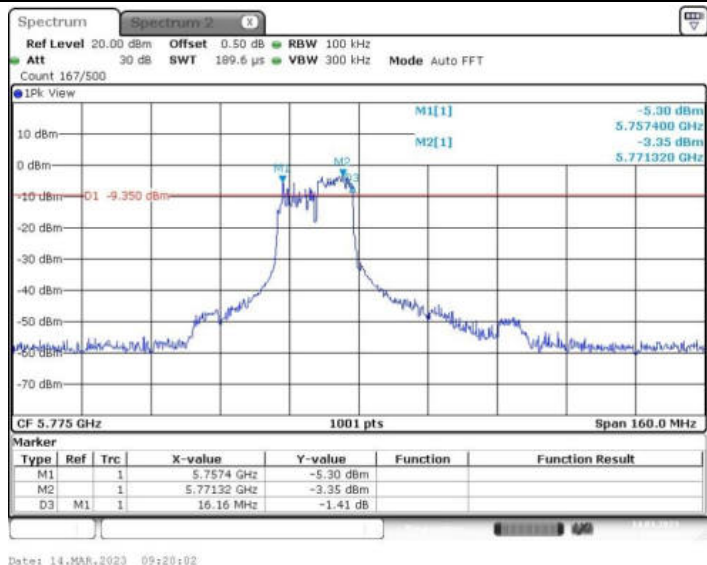
11AX80MIMO_Ant1_5775 242/62
