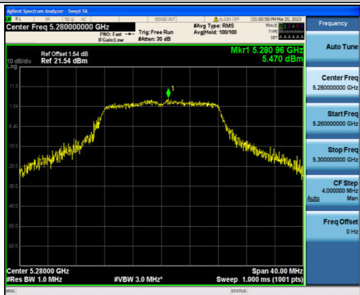
11A_Ant2_5280
