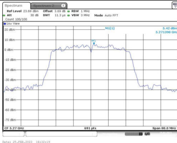
11AC40MIMO_Ant2_5270
