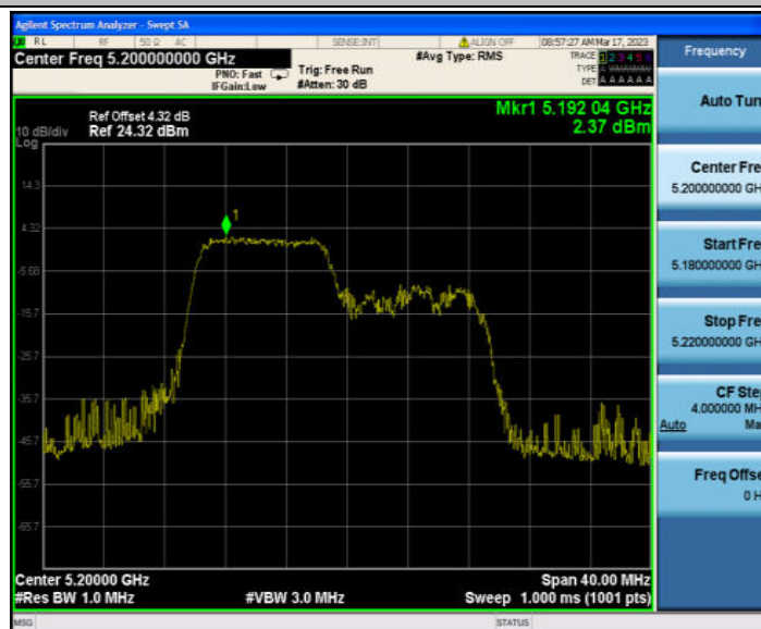
11AX20MIMO_Ant1_5200 242/61
