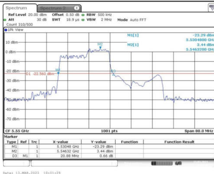
11AX40MIMO_Ant2_5550 106/54
