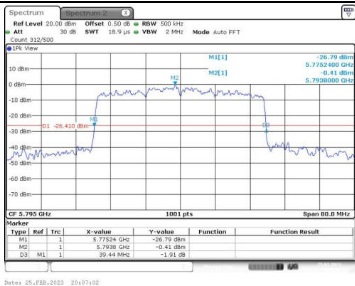
11AX40MIMO_Ant2_5795 484/65
