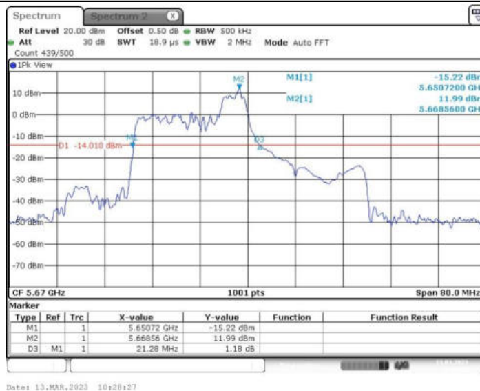
11AX40MIMO_Ant2_5670 52/40
