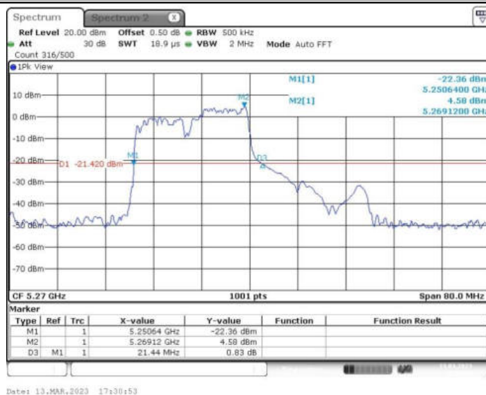
11AX40MIMO_Ant2_5270 106/54
