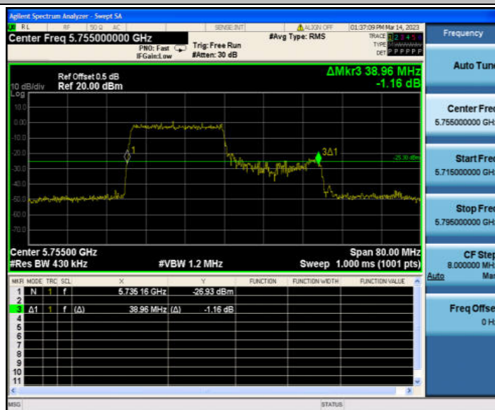
11AX40MIMO_Ant1_5755 484/65
