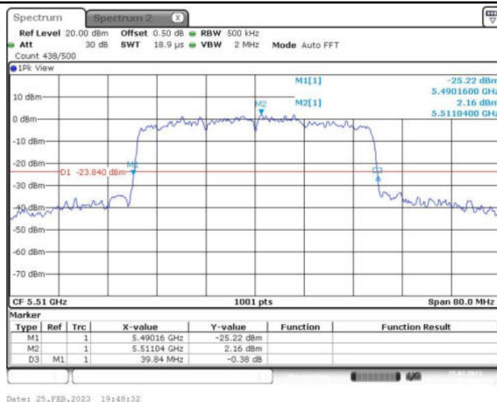
11AX40MIMO_Ant2_5510 484/65
