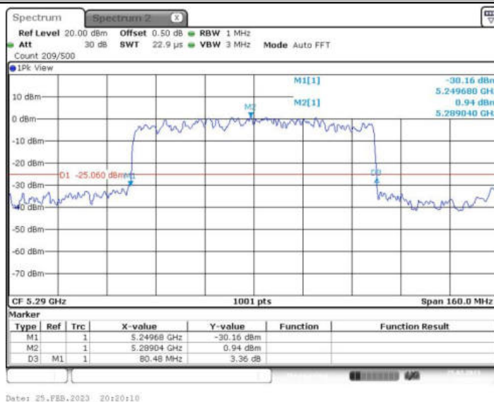
11AX80MIMO_Ant2_5290 996/67
