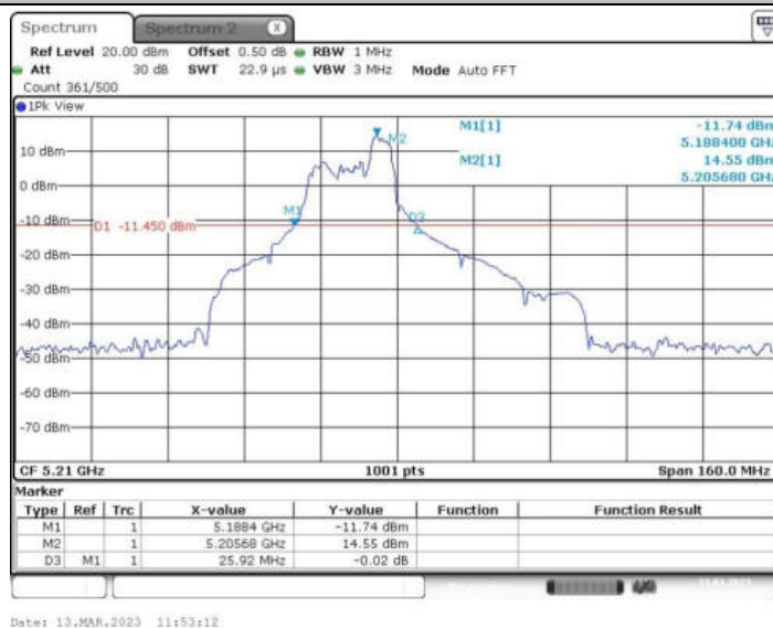
11AX80MIMO_Ant2_5210 52/44
