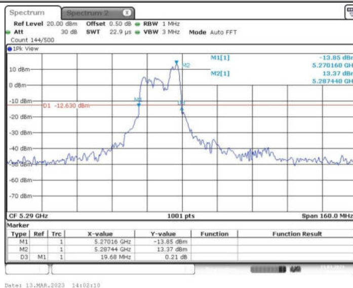
11AX80MIMO_Ant2_5290 52/44
