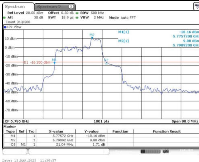
11AX40MIMO_Ant2_5795 52/40
