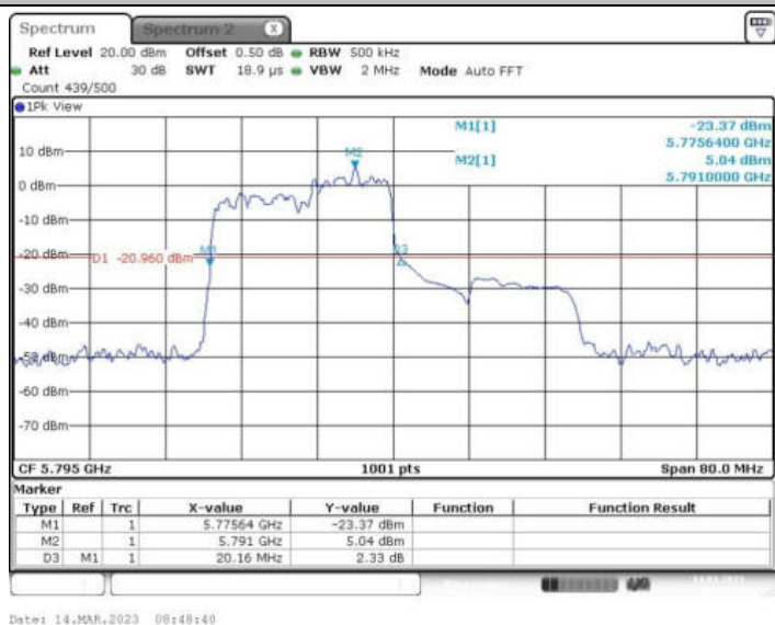
11AX40MIMO_Ant2_5795 106/54
