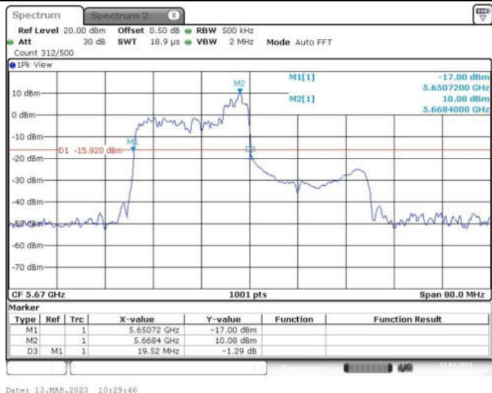
11AX40MIMO_Ant1_5670 106/54
