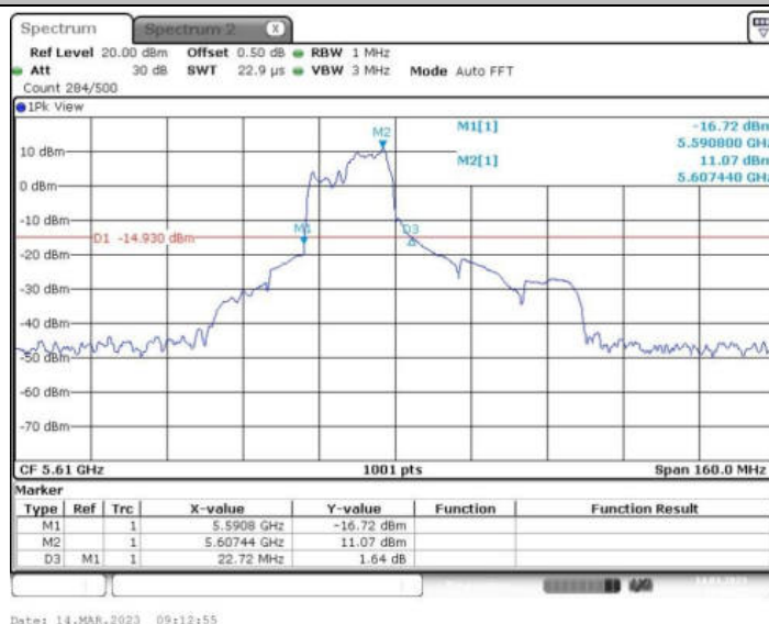
11AX80MIMO_Ant1_5610 106/54
