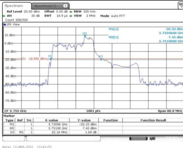
11AX40MIMO_Ant1_5755 106/54
