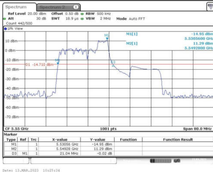
11AX40MIMO_Ant2_5550 52/40
