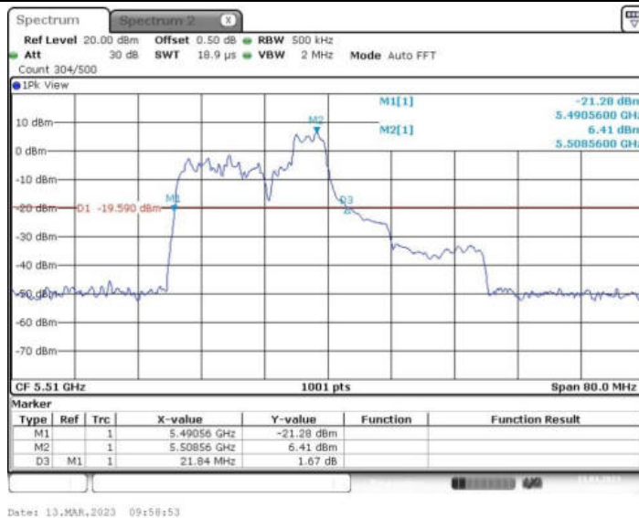
11AX40MIMO_Ant1_5510 106/54
