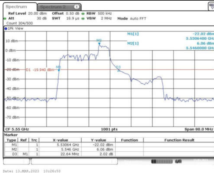
11AX40MIMO_Ant1_5550 106/54
