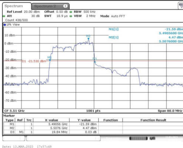
11AX40MIMO_Ant2_5510 106/54
