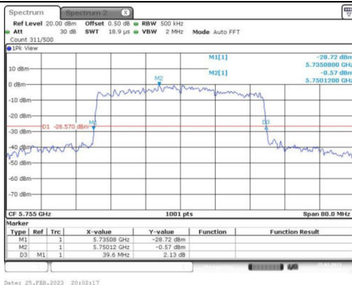
11AX40MIMO_Ant2_5755 484/65
