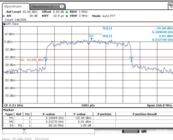
11AX80MIMO_Ant1_5210 996/67
