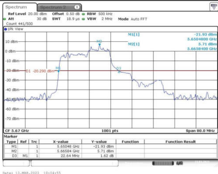
11AX40MIMO_Ant2_5670 106/54
