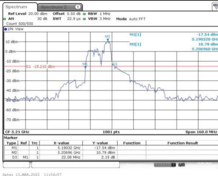
11AX80MIMO_Ant1_5210 106/54
