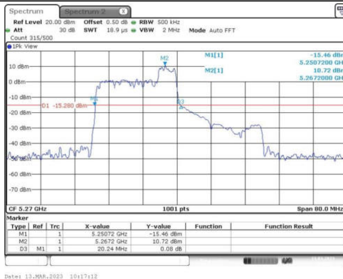
11AX40MIMO_Ant2_5270 52/40
