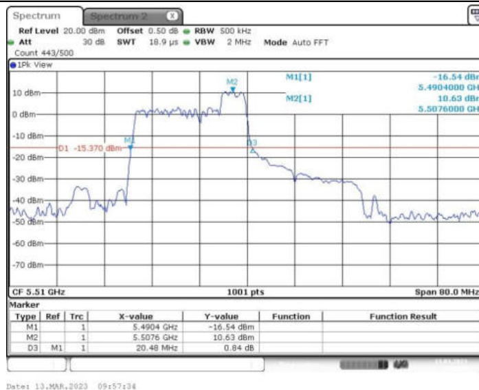
11AX40MIMO_Ant2_5510 52/40
