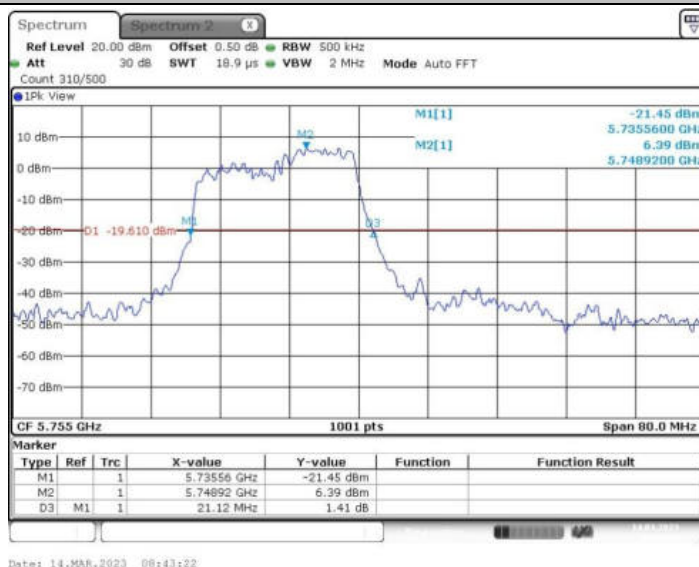
11AX40MIMO_Ant2_5755 106/54
