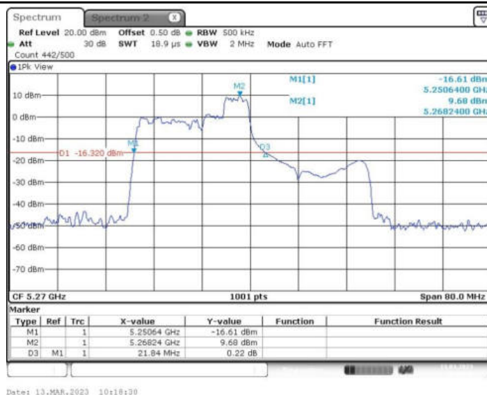
11AX40MIMO_Ant1_5270 106/54
