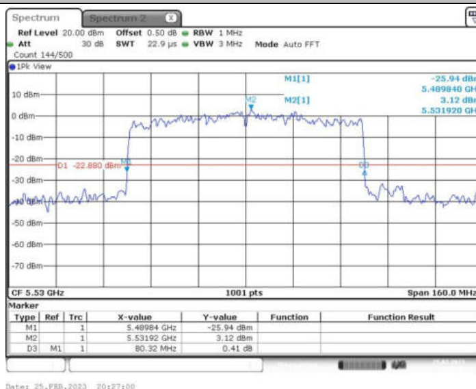
11AX80MIMO_Ant2_5530 996/67
