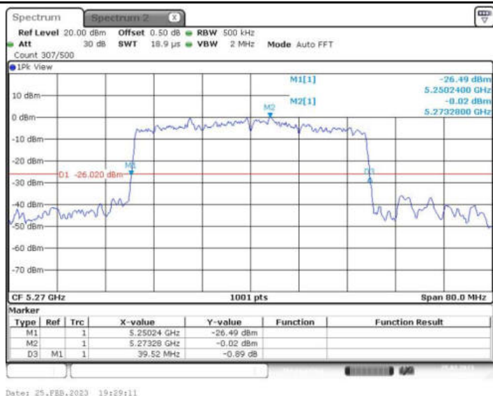
11AX40MIMO_Ant2_5270 484/65
