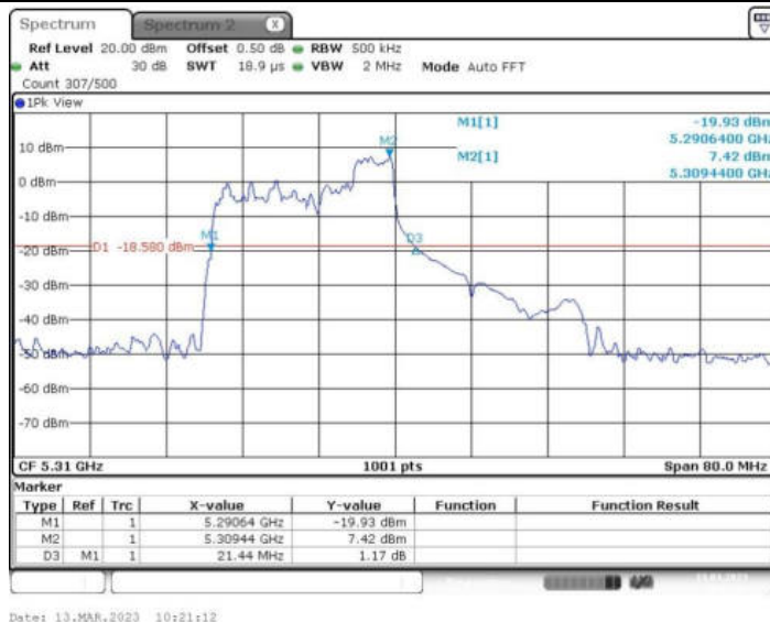
11AX40MIMO_Ant1_5310 106/54
