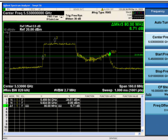
11AX80MIMO_Ant1_5530 996/67
