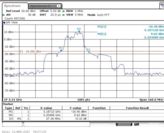
11AX80MIMO_Ant2_5210 106/54
