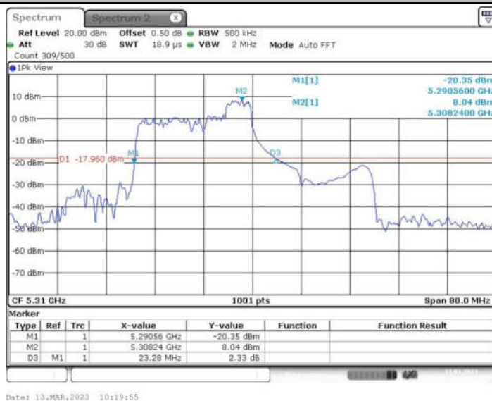
11AX40MIMO_Ant2_5310 52/40
