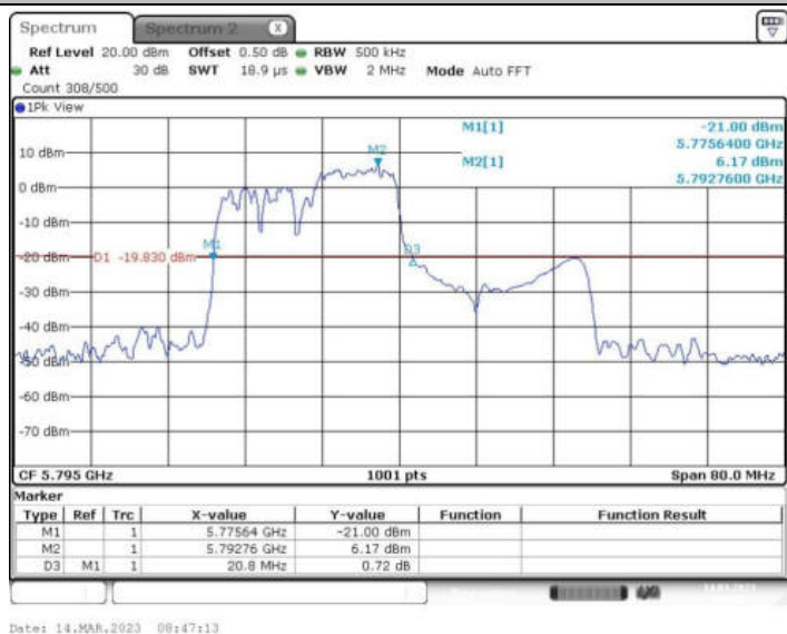
11AX40MIMO_Ant2_5795 106/54
