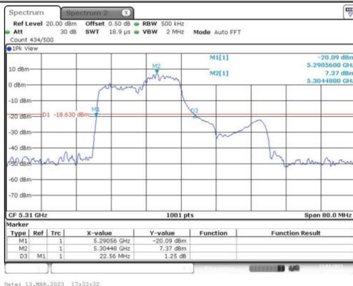
11AX40MIMO_Ant2_5310 106/54
