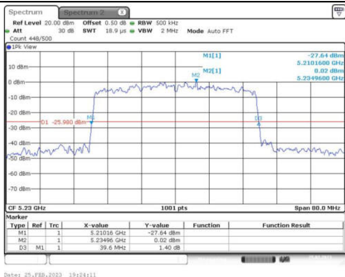
11AX40MIMO_Ant2_5230 484/65
