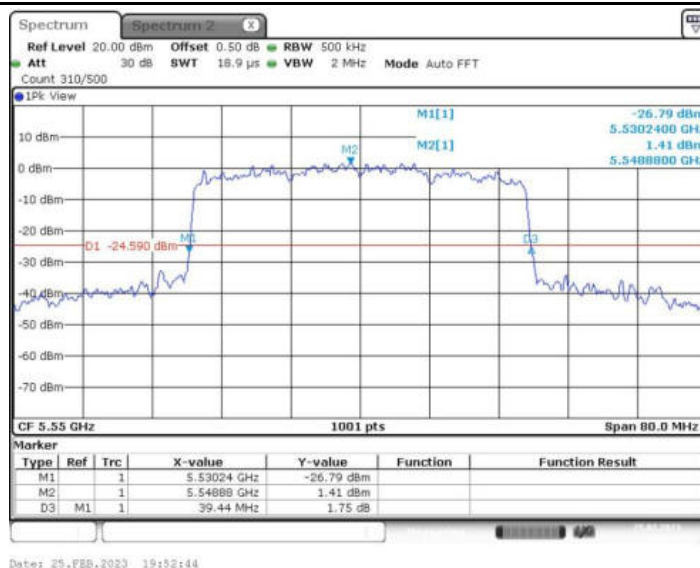
11AX40MIMO_Ant2_5550 484/65
